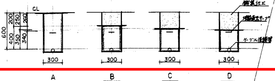
標準埋設断面図 S=1:20
