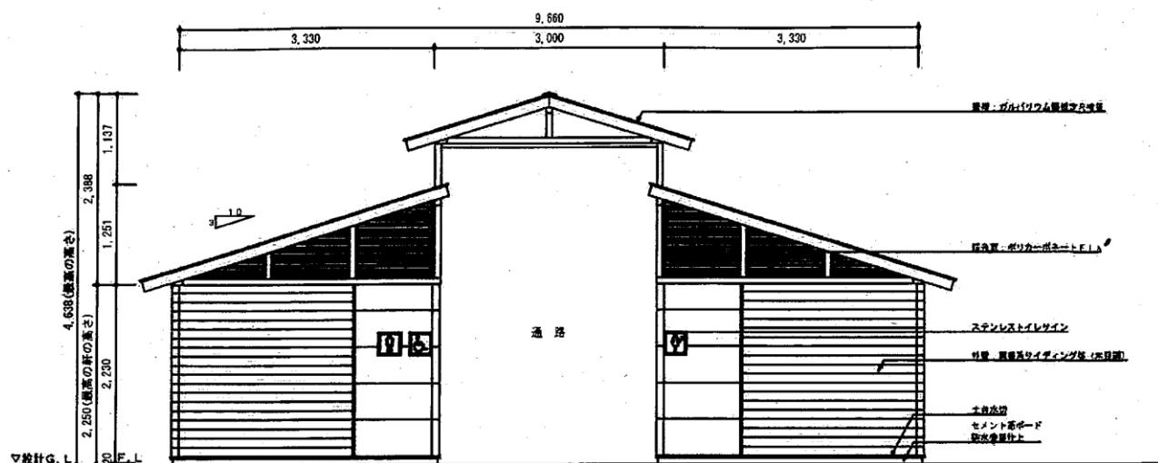
A面立面図 S=1/80
