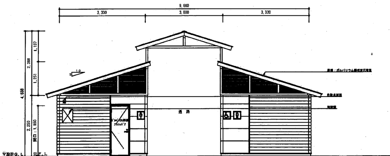
C面立面図 S=1/80
