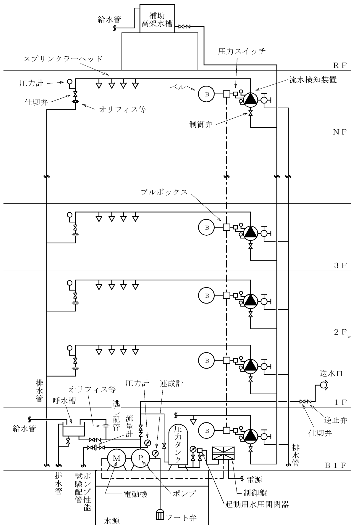
別図－Ⅰ 閉鎖型スプリンクラー設備の配管系統例
