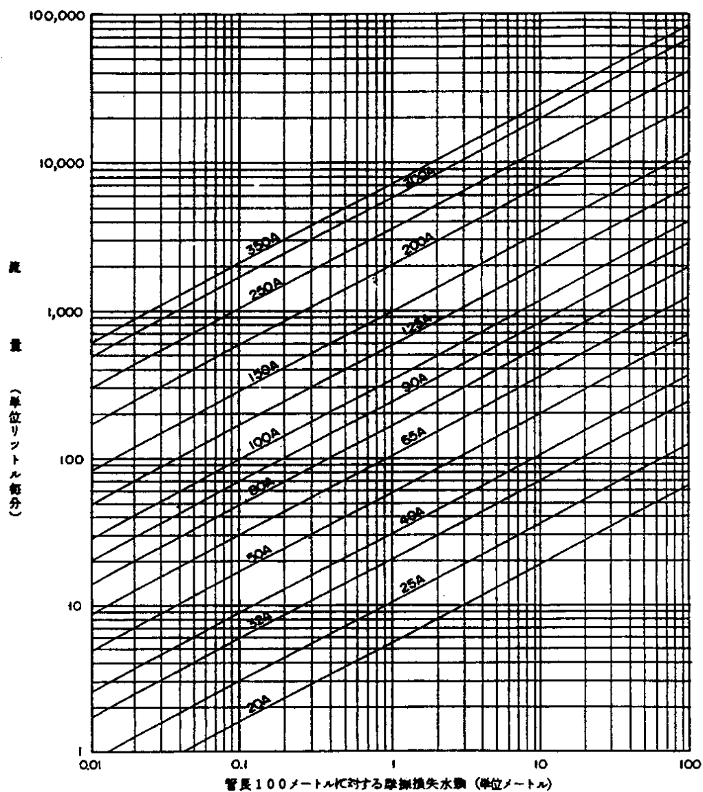
第4-5-15図 溶融亜鉛めっきを施さない配管のうち乾式の部分に用いる摩擦損失水頭線図
