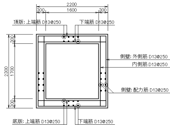
第4-17-4図 2KLの場合の断面図
