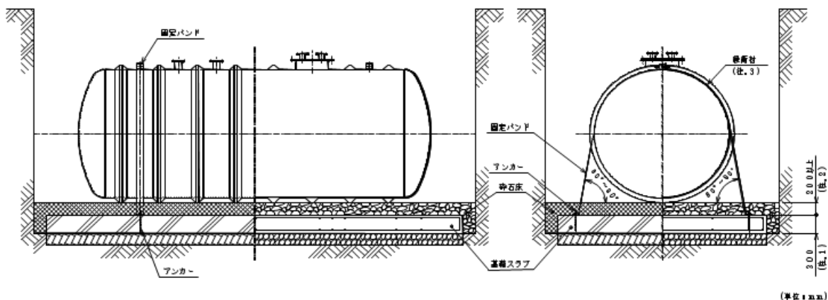
第4-18.2-1図（その1） 6号砕石等又はクラッシャランを用いる場合の砕石床施工図
