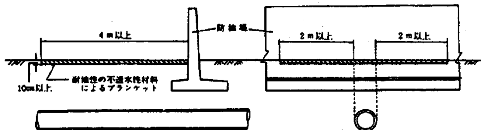
第4-16-15図 ブランケットの設置
