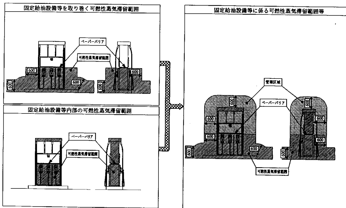
第4-7-8図 ベーバーバリアを設置した地上式固定給油設備の例2
