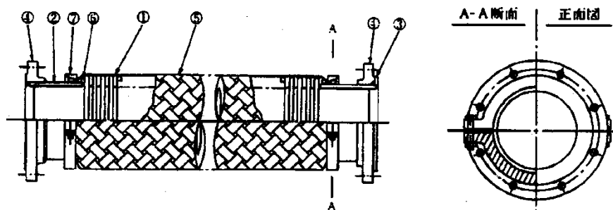
第4-15-1図 フレキシブルメタルホース構造図例
