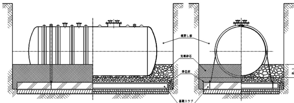
第 4-18.2-1 図（その3） 6号碎石等又はクラッシャランを用いる場合の充填碎石施工図
