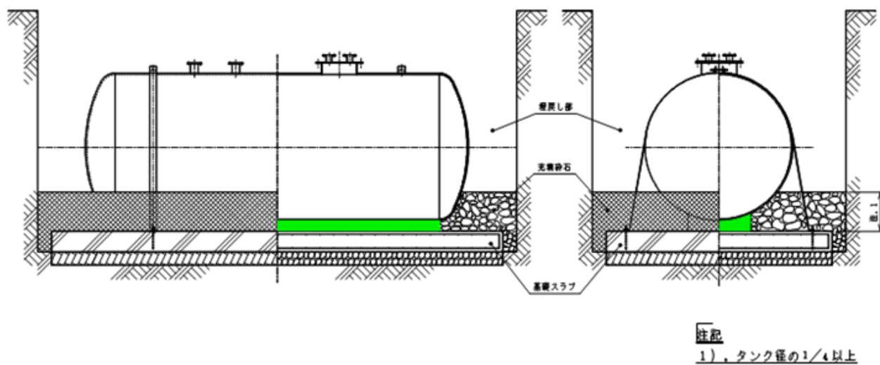
第4-18.2-3図（その2） 発泡剤を用いる場合の充填碎石施工図
