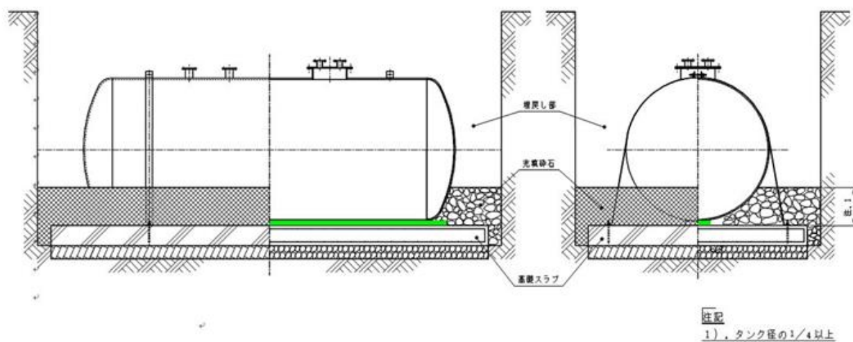
第4-18.2-2図（その2） ゴム板を用いる場合の充填砕石施工図 （支持砕石は第第4-18.2-1図（その2）のとおり施工されているものとする）
