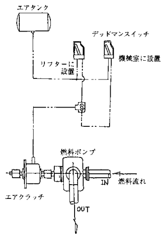
デッドマン・コントロールシステム系統図
