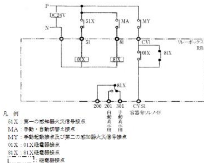
図2 継電器盤（1回線用）の回路例
