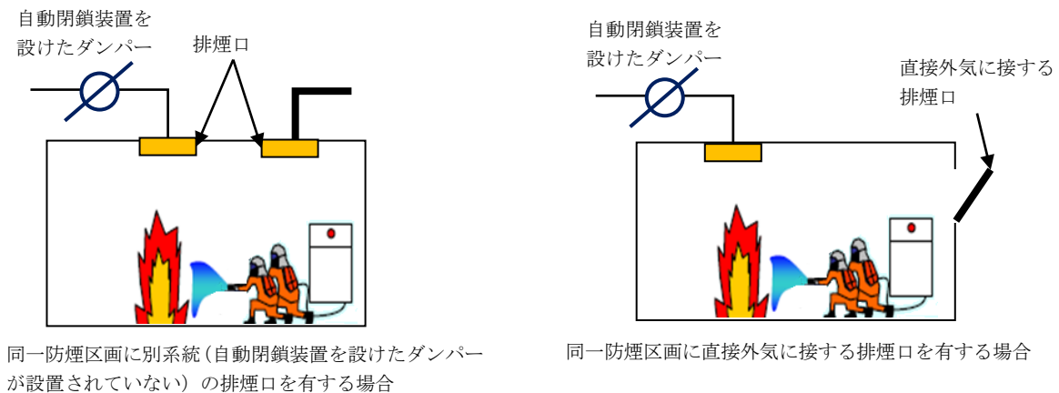
第30－3図 自動閉鎖装置を設けたダンパーを設置して差し支えない場合の例
