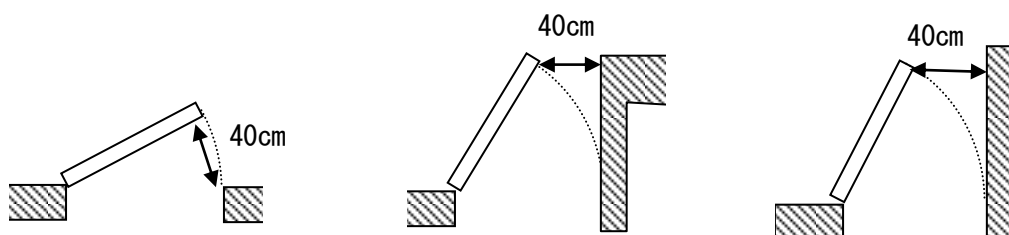
第30－6図 遮煙開口部の開口幅
