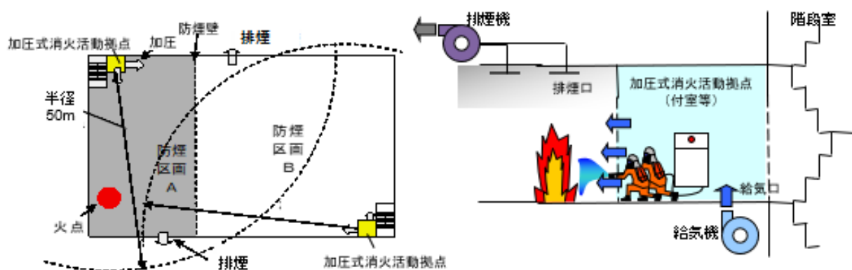
第30－Ⅰ図 加圧防排煙設備の概要
