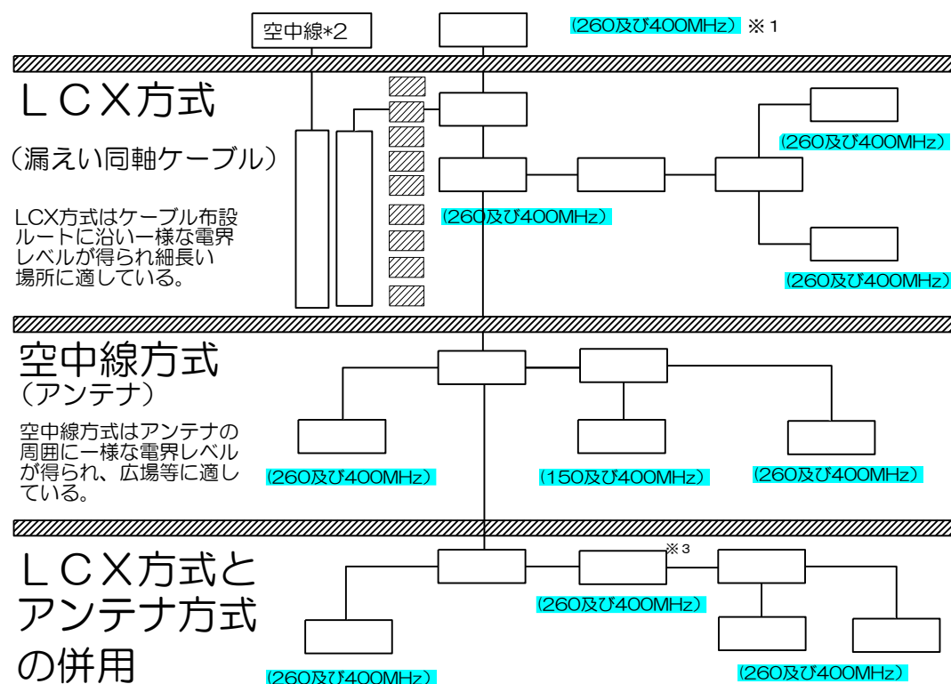
無線通信補助設備の方式
