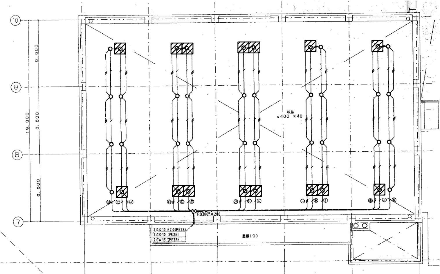
体育館 3 階平面図
