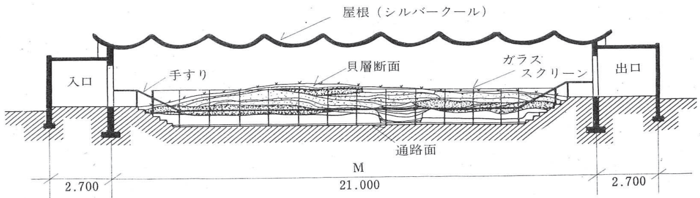
3 施設断面図 縦断面図
