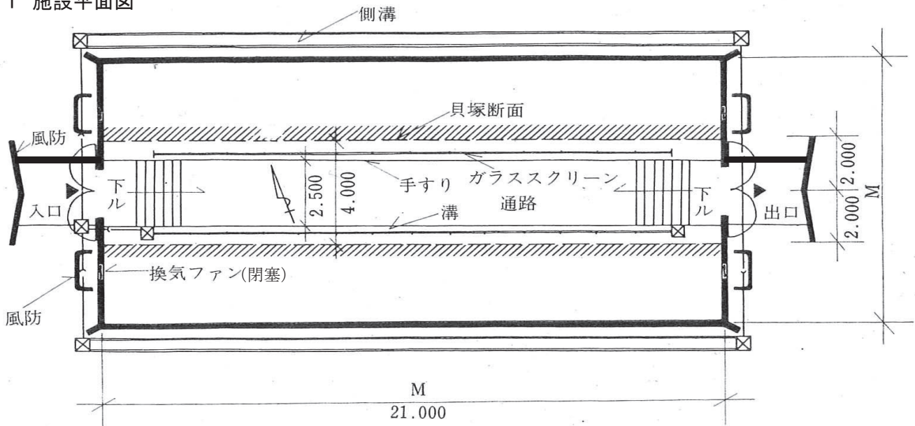
1 施設平面図
