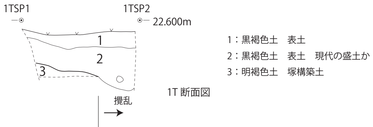
試掘 1 トレンチ断面図
