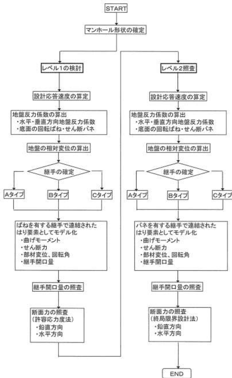
図 12.3.4 組立式マンホールの耐震設計フロー
