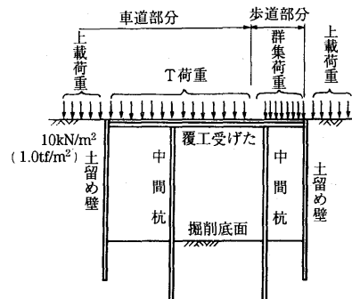
図 7.5.1 活荷重の載荷状況
