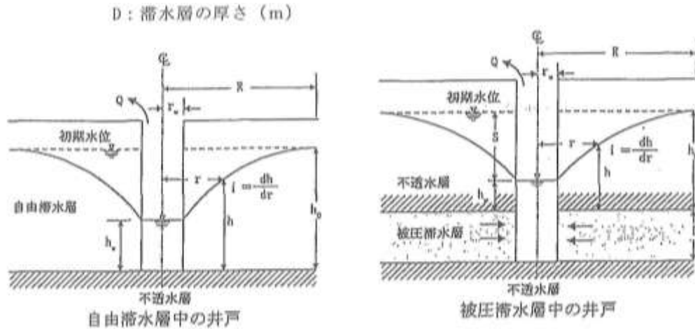
図 11.4.4 滞水条件による井戸
