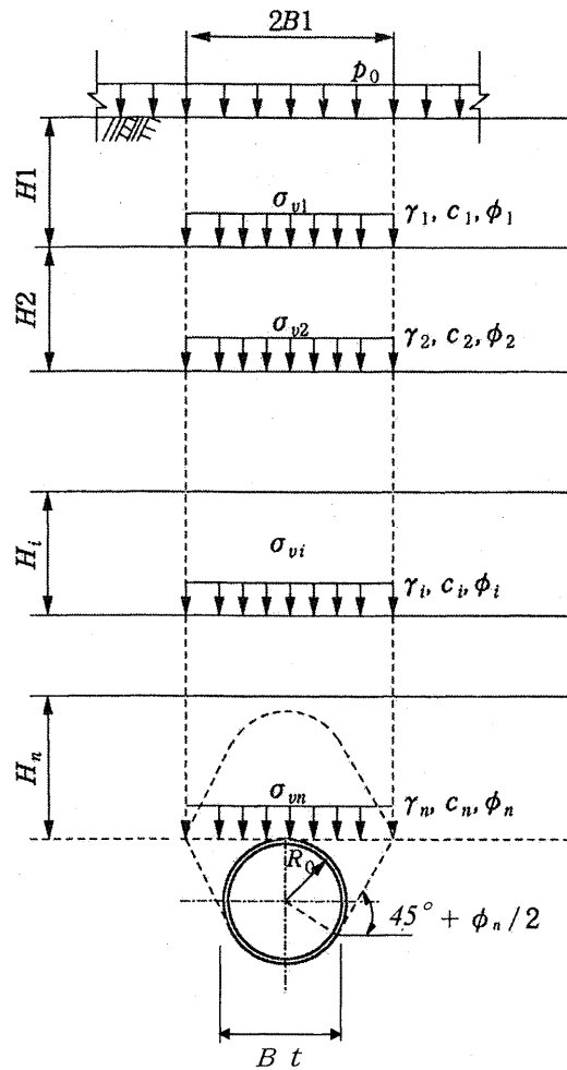
図 8.3.4 多層地盤における緩み土圧
