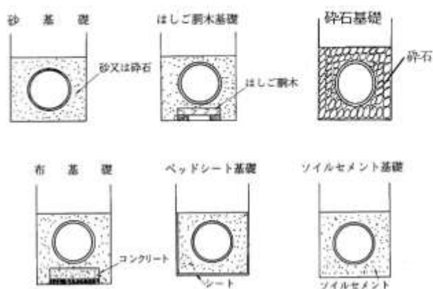
図 4.6.2 可とう性管きよの基礎の種類
