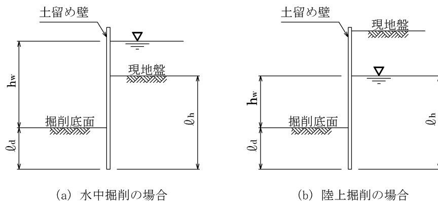
図 7.8.2 パイピングの検討
