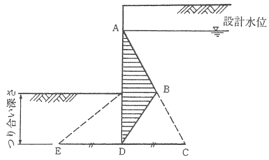
図 7.6.5 水圧分布
