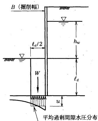
図 7.8.1 ボイリングの検討方法
