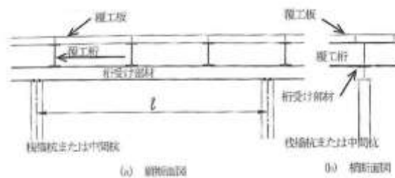
図 7.10.5 桁受け部材の支間（溝形鋼の場合）
