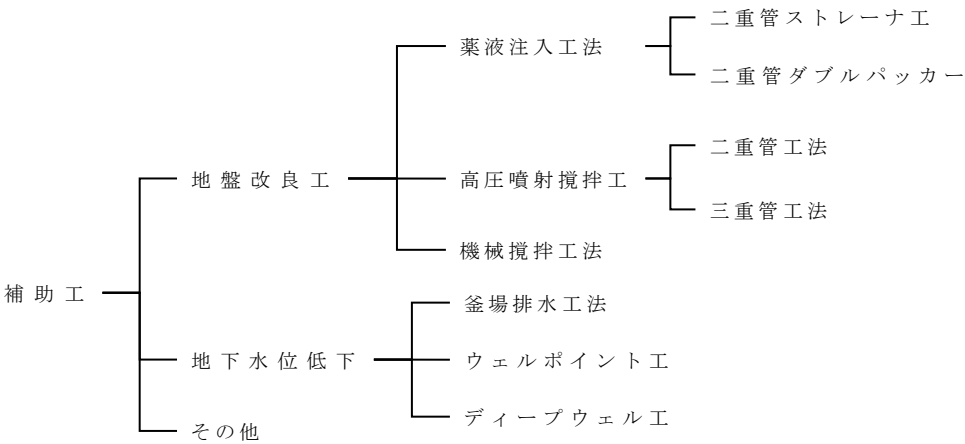
図 11.1.1 補助工法の種類
