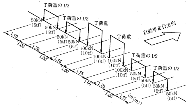
図 7.10.1 T 荷重の載荷配列
