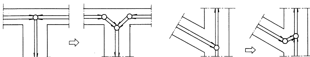
図 4.5.3 管きよが曲折する場合
