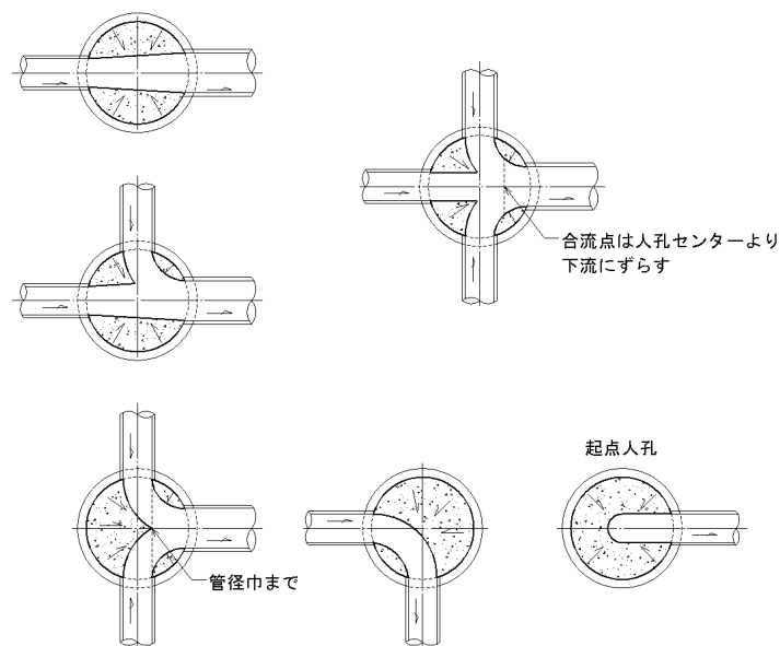
図 5.7.1 インバート・標準図
