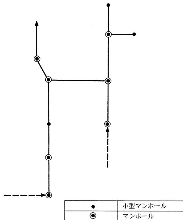
図 5.11.1 小型マンホールの設置例
