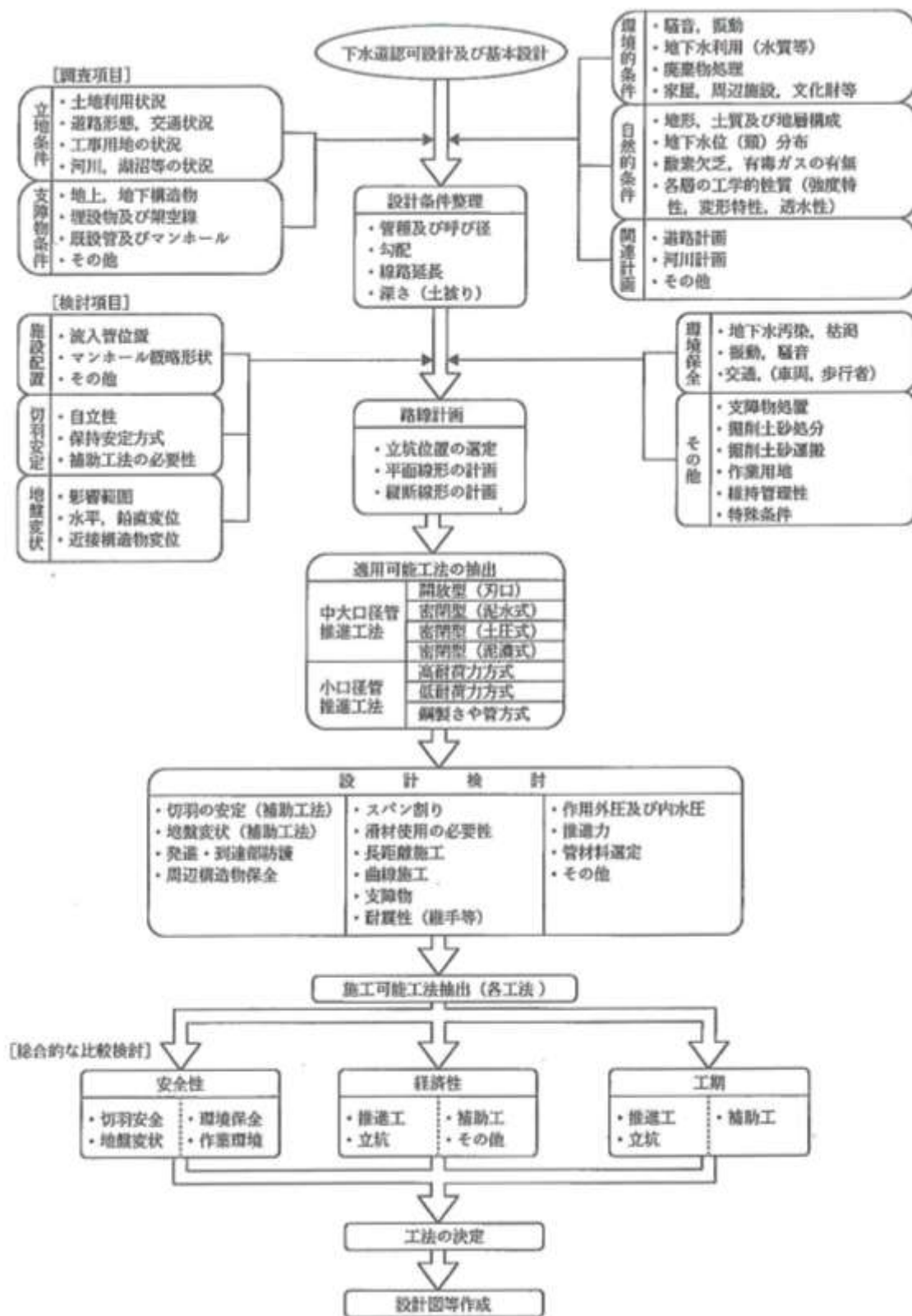
図 8.2.1 推進工法の選定フロー
