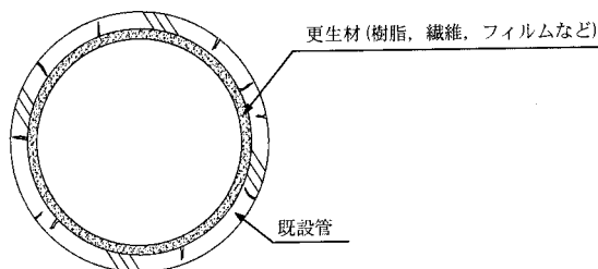
図 10.2.1 自立管の概念
