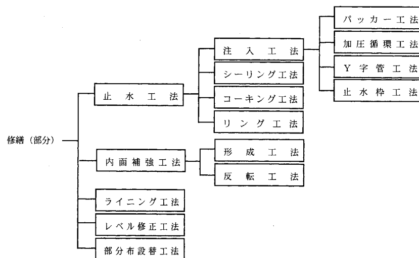
図 10.1.3 修繕工法の分類
