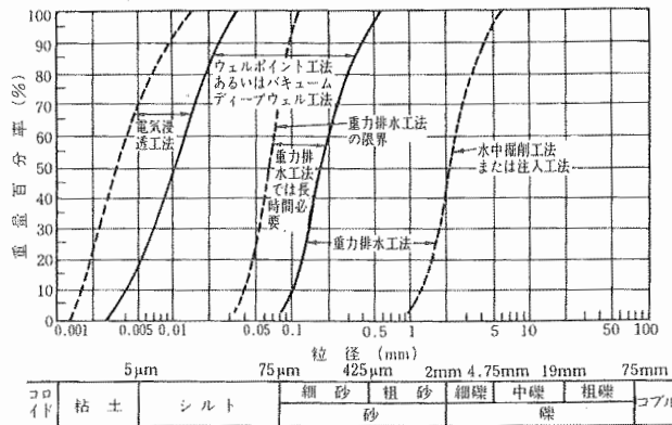
図 11.4.1 各種土質に適用される地下水位低下工法
