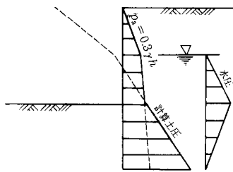
図 7.6.1 粘性土地盤の主働側圧の考え方
