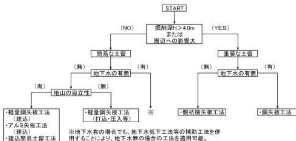
図 7.4.2 土留め工法選定
