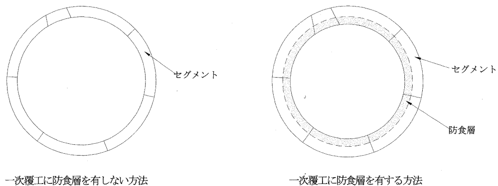
図 9.3.1 下水道トンネル断面図例
