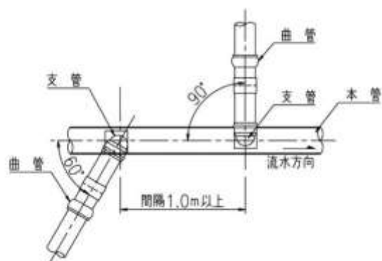
図 6.2.2 取付管間隔の例
