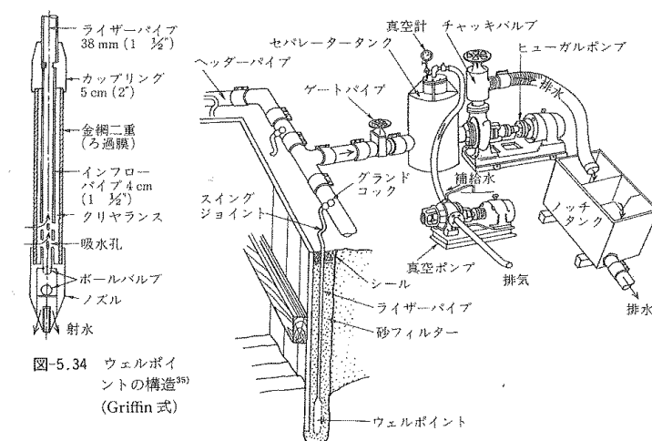
図 11.4.3 ウェルポイント工法設置概要図
