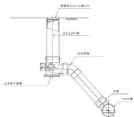
図 6.2.1 取付管の標準配管例
