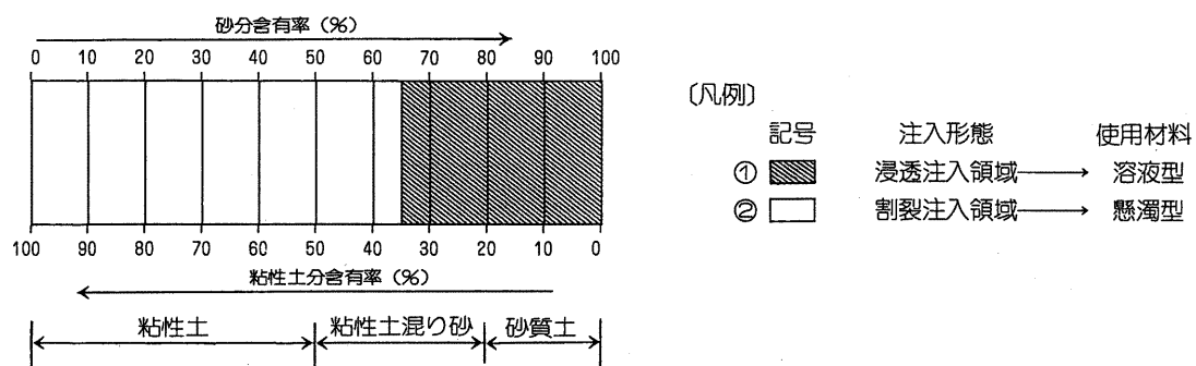
図 11.2.2 粒度と注入形態と材料
