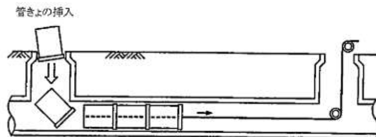
図 10.2.8 鞘管工法の概要図
