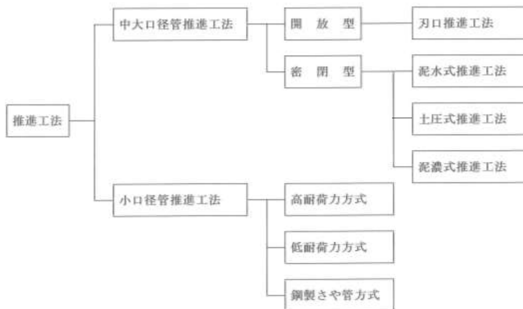
図 8.1.1 推進工法の分類
