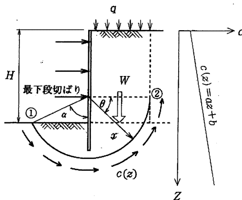
図 7.8.3 ヒービングの検討
