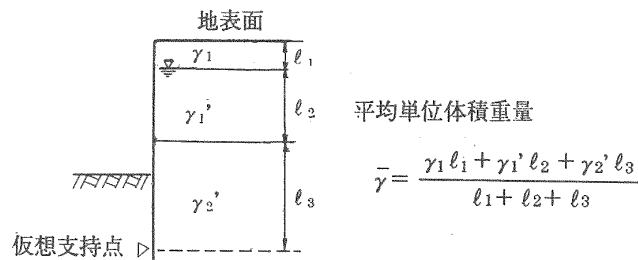
図 7.6.3 土の平均単位体積重量の求め方
