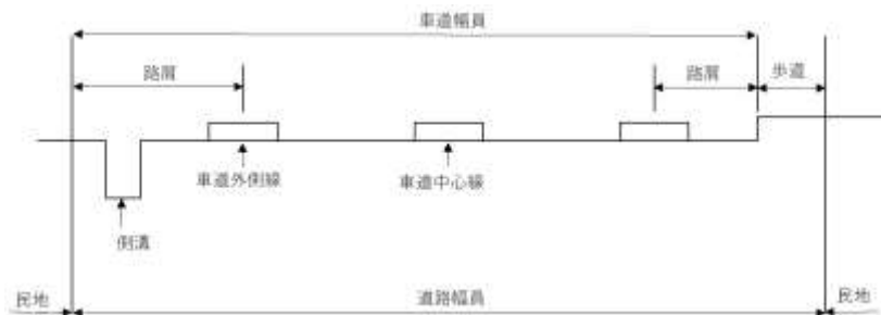
図 5.5.1 車道路幅員
