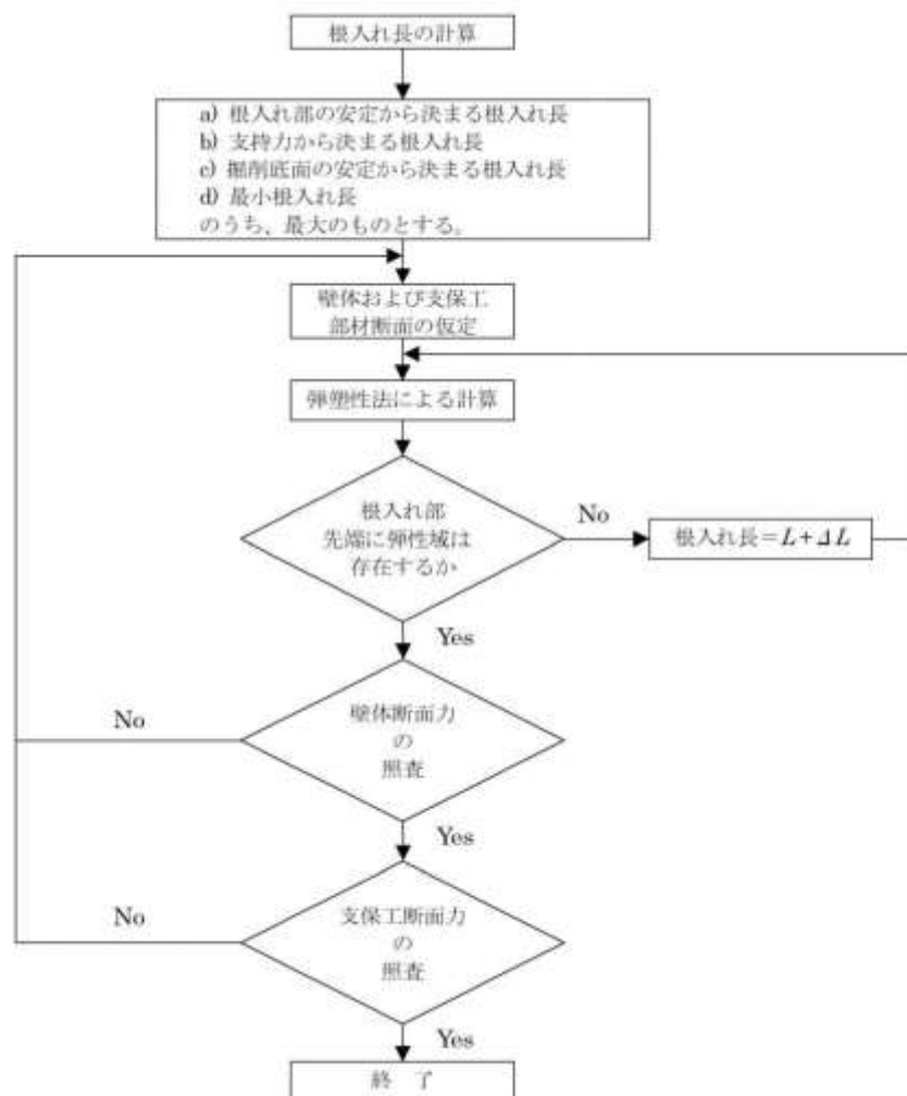
図 7.8.11 根入れ長決定の手順
