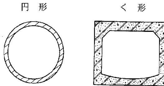
図 4.2.1 管きよ断面の種類
