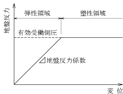
図 7.8.12 地盤バネの特性
