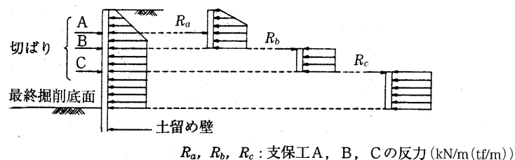
図 7.9.1 慣用法を用いた場合の支保工の設計に用いる荷重(下方分担法)
