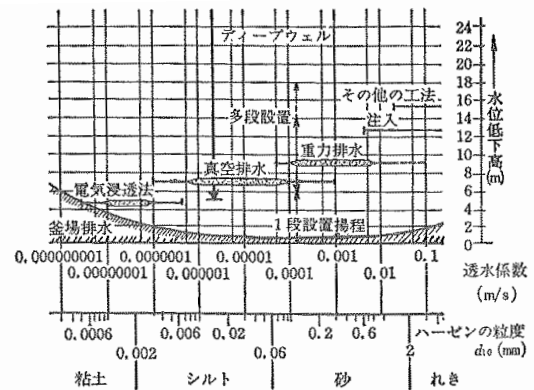
図 11.4.2 各土質に対する排水法
