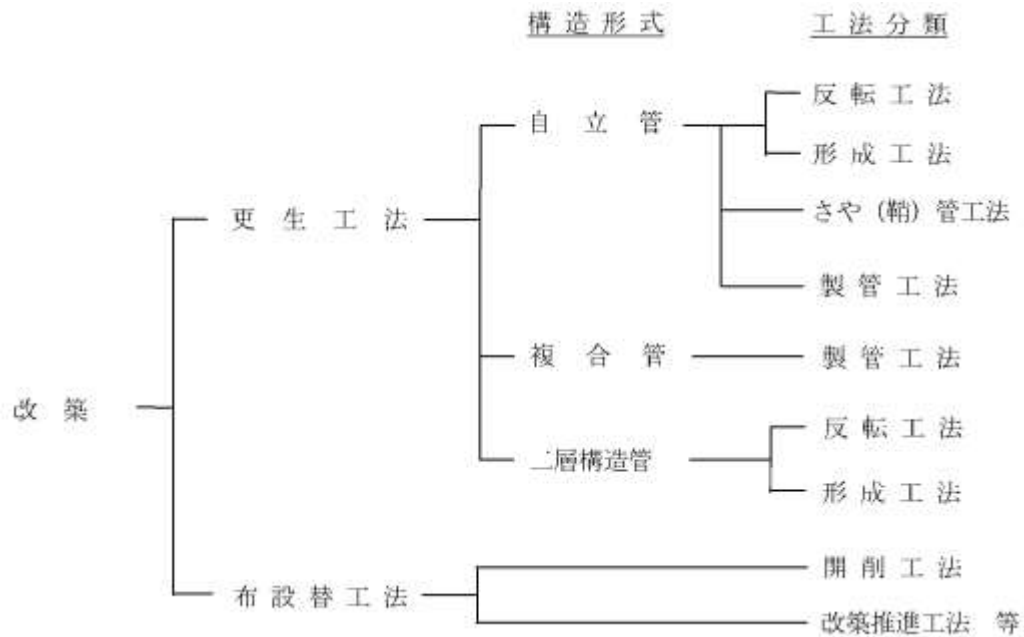
図 10.1.2 改築工法の分類
