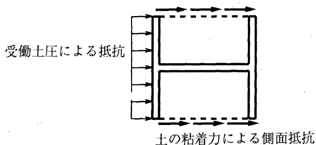
図 7.8.6 親杭の根入れ部の地盤抵抗
