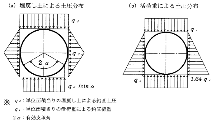
図 4.7.3 土圧分布状態
