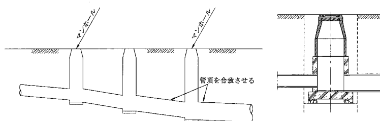
図 4.5.1 管頂接合
