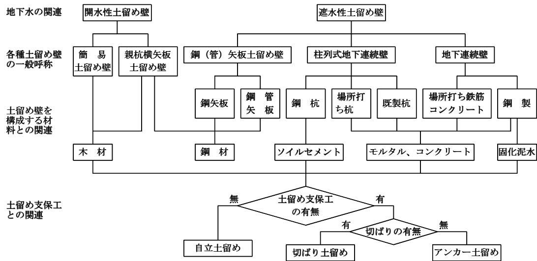
図 7.1.1 土留めの種類と区分
