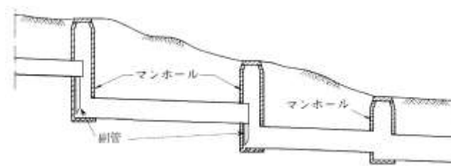
図 4.5.2 段差接合の例
