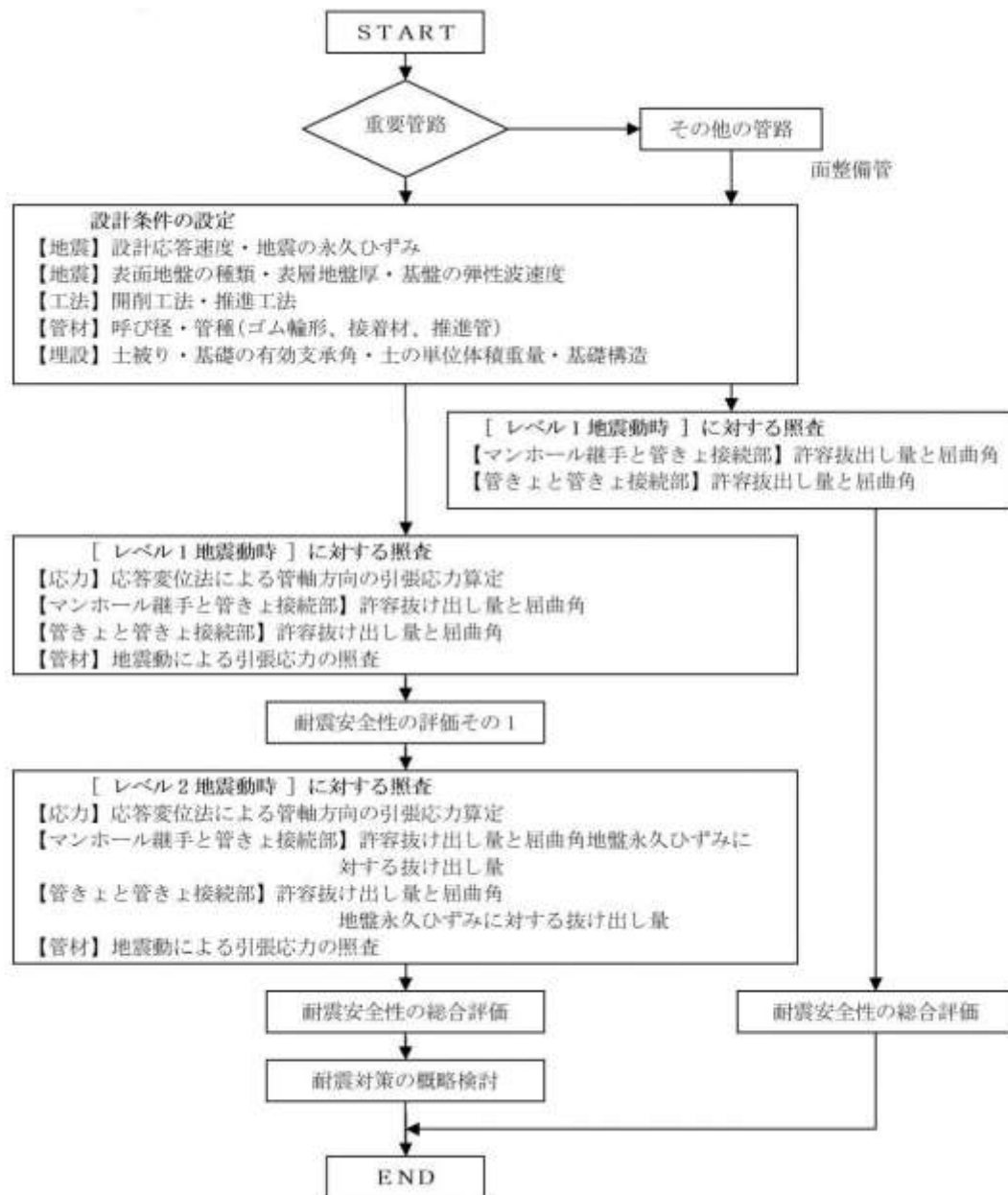
図 12.3.3 塩ビ管の耐震設計フロー
