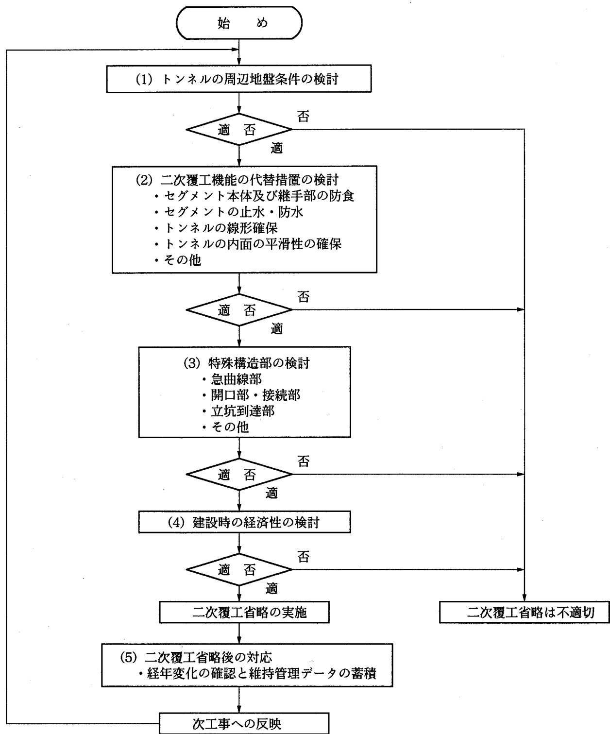
図 9.4.1 二次覆工省略の検討フロー
