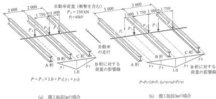
図 7.10.3 覆工受桁と自動車走行方向が平行な場合の載荷方法 出典：トンネル示方書・開削
