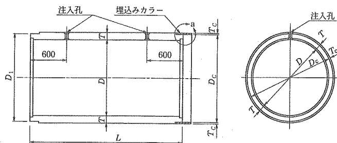
図 8.4.1 標準管の形状
