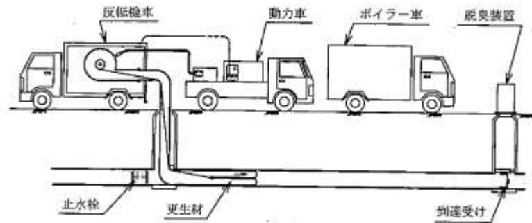
図 10.2.4 反転工法の概要図
