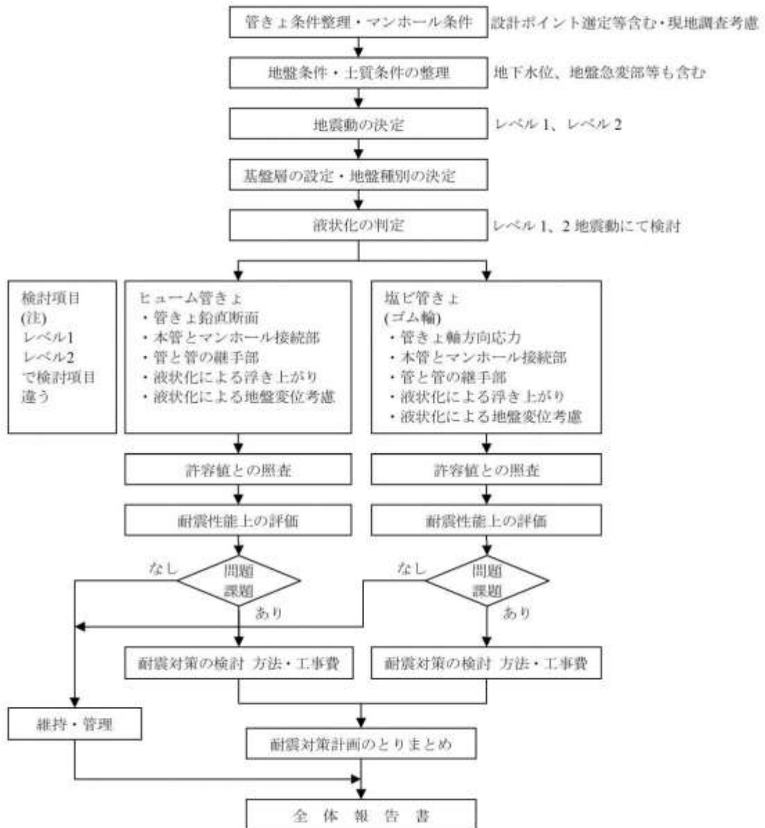
図 12.3.1 耐震設計作業手順(全体的な作業手順)
