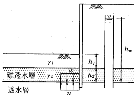
図 7.8.4 盤ぶくれに対する検討
