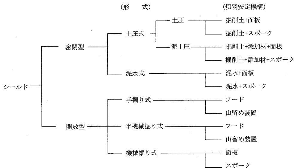
図 9.1.1 推進工法の分類
