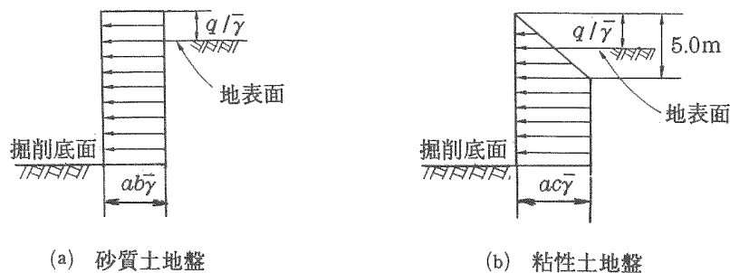
図 7.6.4 地表面での上載荷重がある場合の土圧
