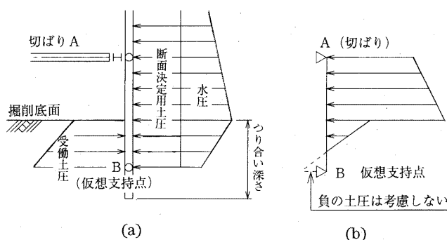
図 7.8.7 鋼矢板の断面計算
