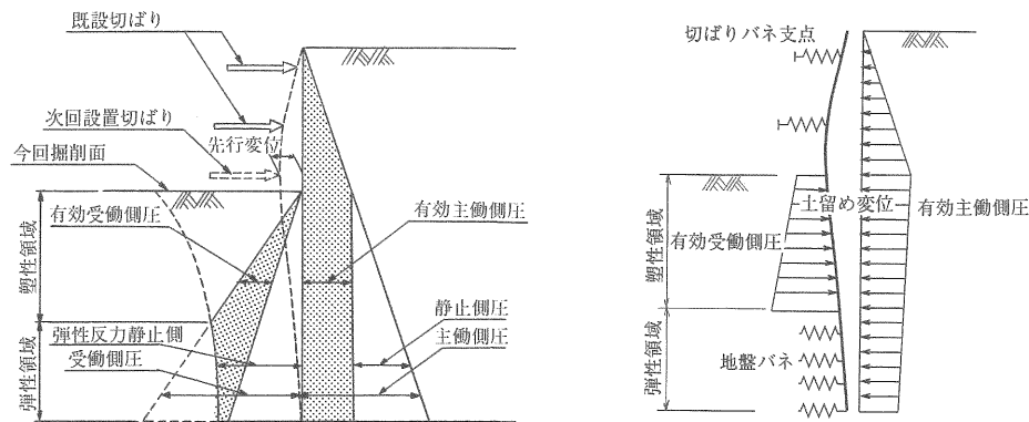
図 7.8.13 側圧、構造系説明図
