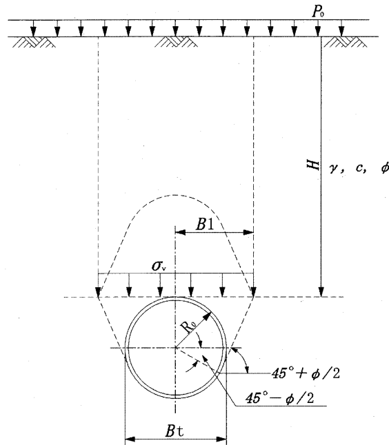
図 8.3.3 均一地盤における緩み土圧
