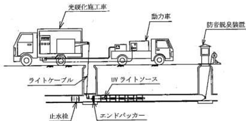
図 10.2.5 形成工法（光硬化タイプ）の概要図
