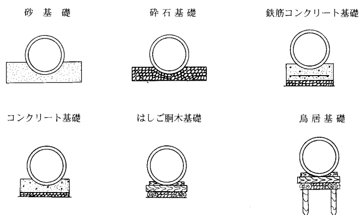
図 4.6.1 剛性管きよの基礎の種類
