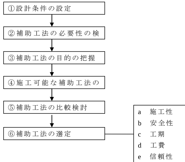
図 11.1.2 補助工法の選定手順
