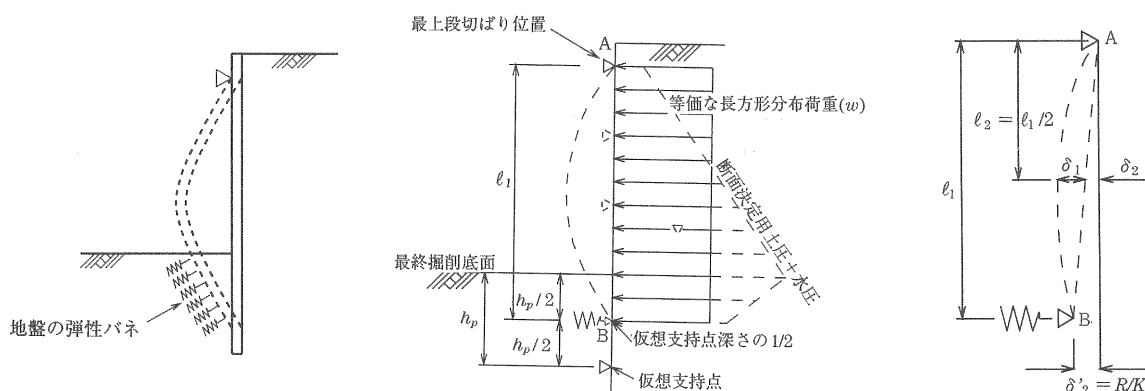
図 7.8.8 鋼矢板変形のモデル化 変位量の求め方
