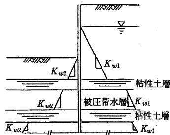
図 7.6.9 上層地盤に粘性土層がある場合
