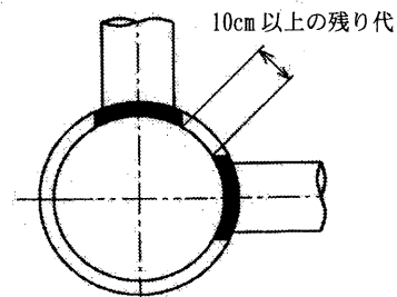
図 5.3.1 削孔間隔
