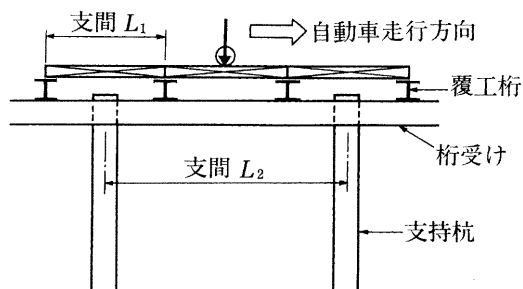
図 7.10.2 覆工受桁と自動車走行方向が直角な場合の部材の支間
