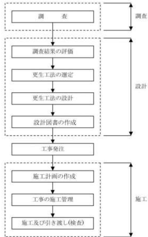
図 10.2.9 管きょ更生工法の調査・設計・施工手順
