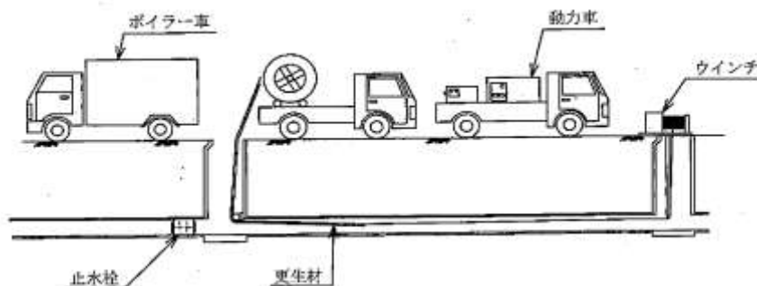
図 10.2.6 形成工法（熱形成タイプ）の概要図
