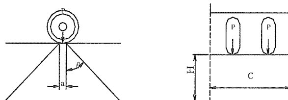
図 8.3.1 輪荷重の分布
