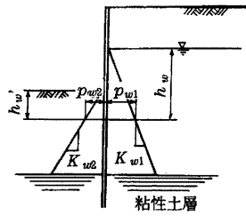
図 7.6.7 砂質土地盤の水圧
