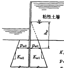
図 7.6.8 下層地盤に粘性土層がある場合
