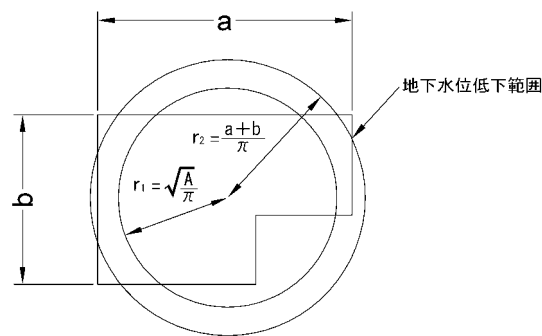
図 11.4.5 仮想井戸の半径
