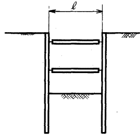
図 7.8.14 切ばりの長さ
