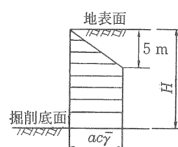
(b) 粘性土地盤の土圧分布
