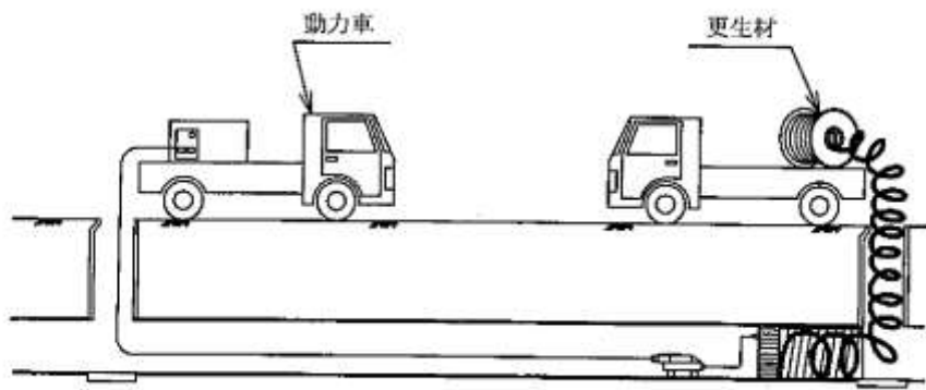
図 10.2.7 製管工法の概要図
