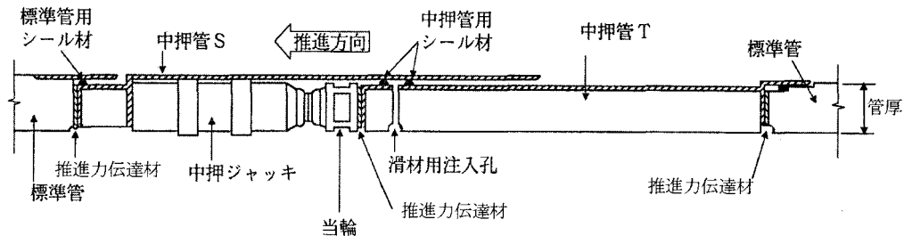
図 8.3.5 中押管及び中押ジャッキの配置例
