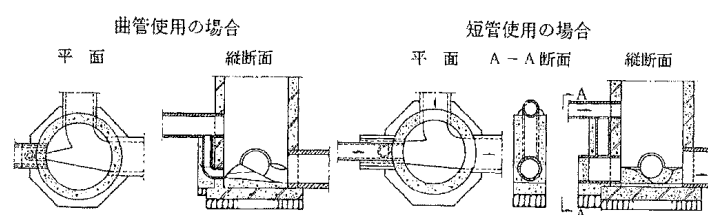
図 5.10.1 外副管付きマンホールの例
