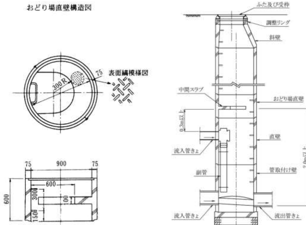
図 5.8.1 中間スラブ設置例(マンホール深さ：5.0m 以上の場合)
