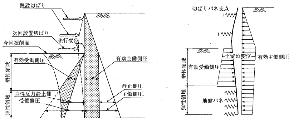
図 7.6.6 弾塑性法の概念図
