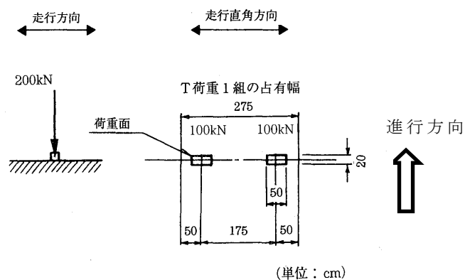
図 7.5.2 T 荷重
