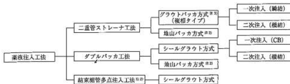
図 2-5 現在使用されている注入工法の分類
