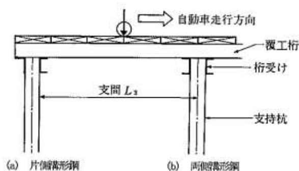
図 7.10.4 覆工受桁と自動車走行方向が平行な場合の部材の支間 出典：トンネル示方書・開削
