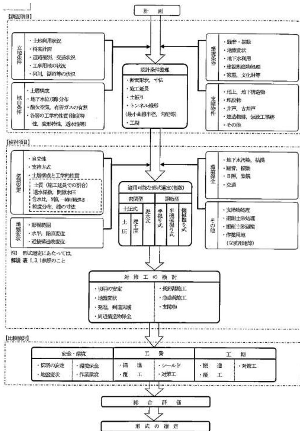
図 9.2.1 形式選定フロー図例
