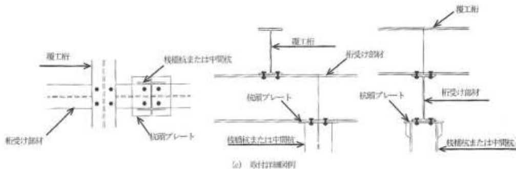
図 7.10.6 桁受け部材の支間（H形鋼の場合）
