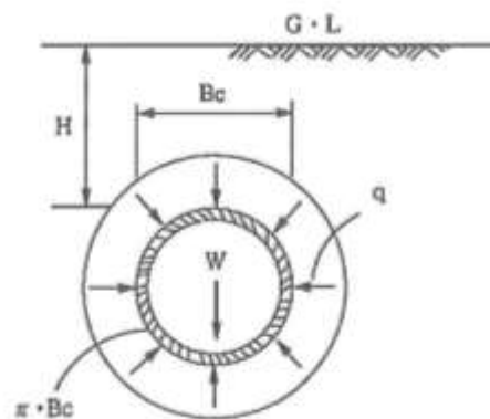
図 8.4.3 推進諸抵抗
