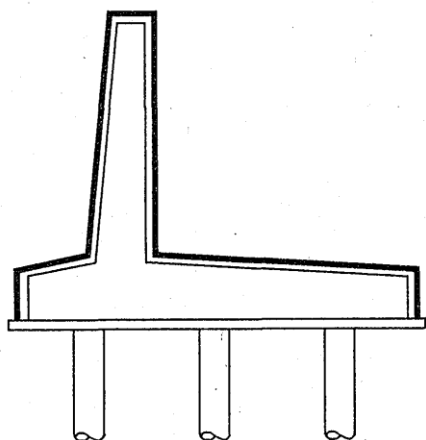
図－1 擁壁
