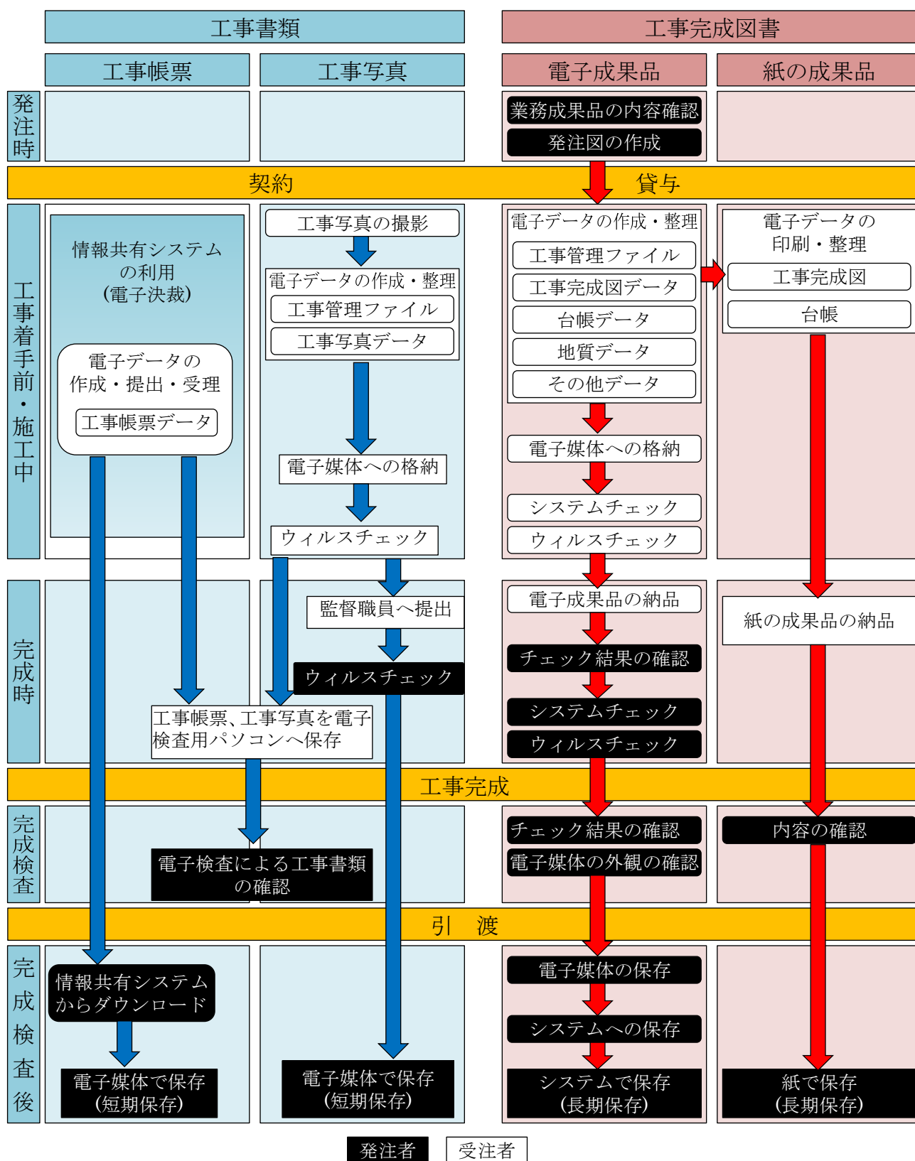
図 2-2 土木工事における電子納品・電子検査の流れ（情報共有システムを利用する場合）
