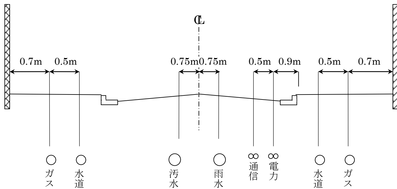
幅員 9.00m 以上 12.00m 未満
