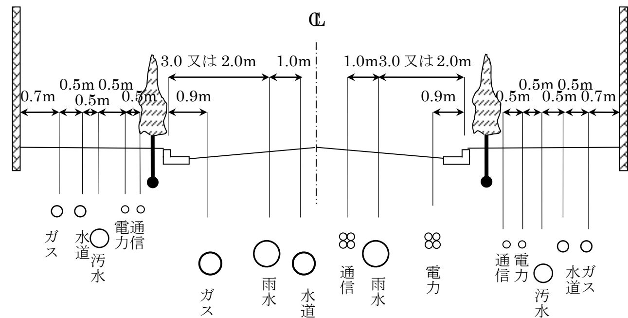
幅員 12.00m 以上 18.00m 未満(その 2)
