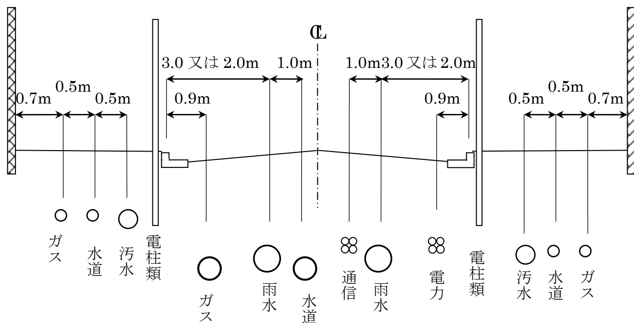
幅員 12.00m 以上 18.00m 未満(その 1)
