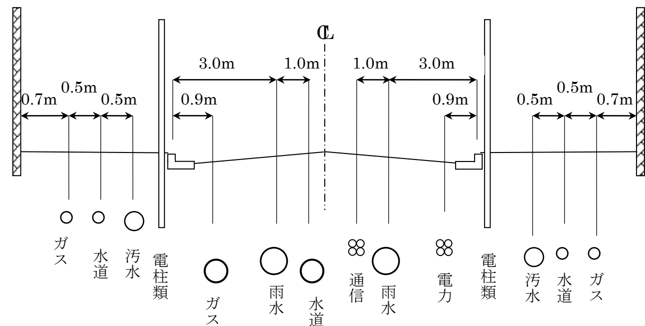
幅員 18.00m 以上(その 1)
