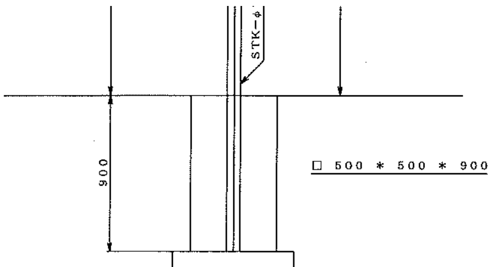
基礎構造略図
