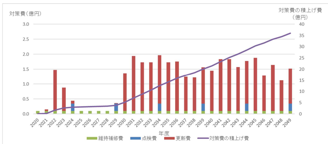
図 3 年度別予防保全時の対策費用（平準化後）
