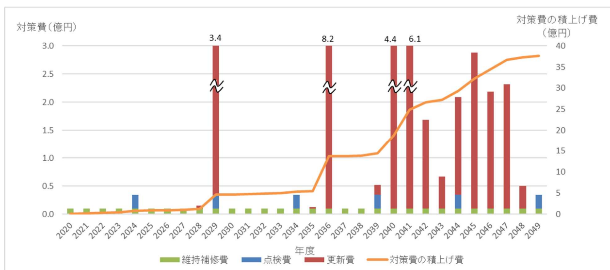
図2 年度別事後保全時の対策費用（平準化前）
