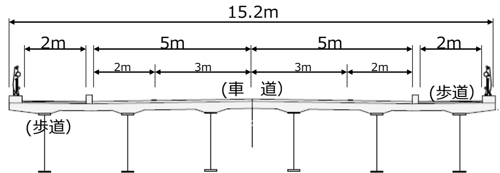
完成後 (断面図)
