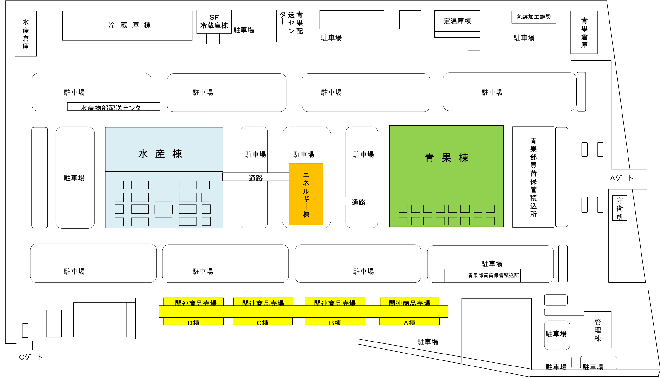
●千葉市地方卸売市場内施設配置図
