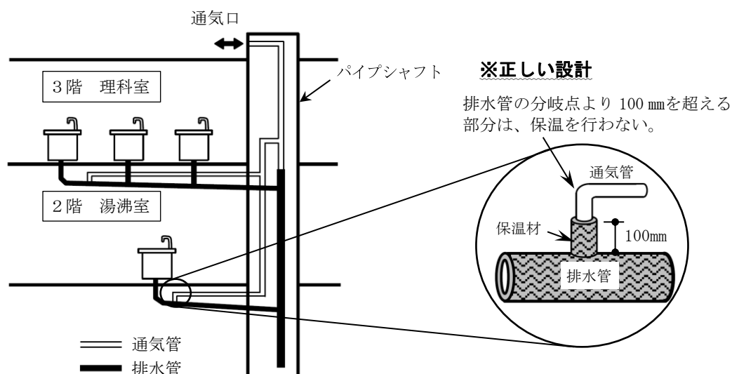
※排水管と通気管の概略図
