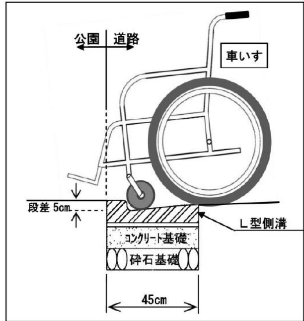
断面図（南側出入口）
