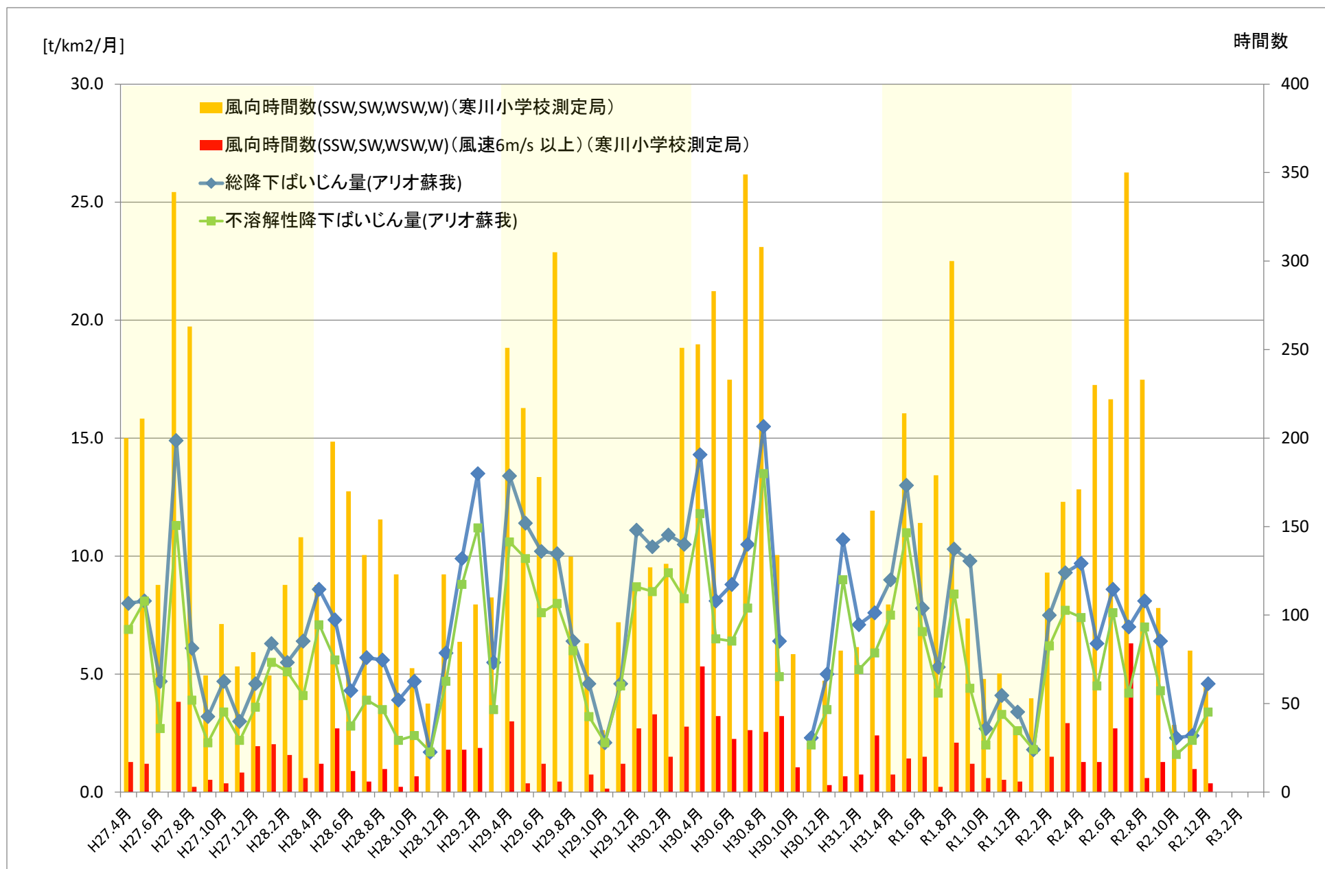
図3 アリオ蘇我における降下ばいじん量測定結果(経月変化)
