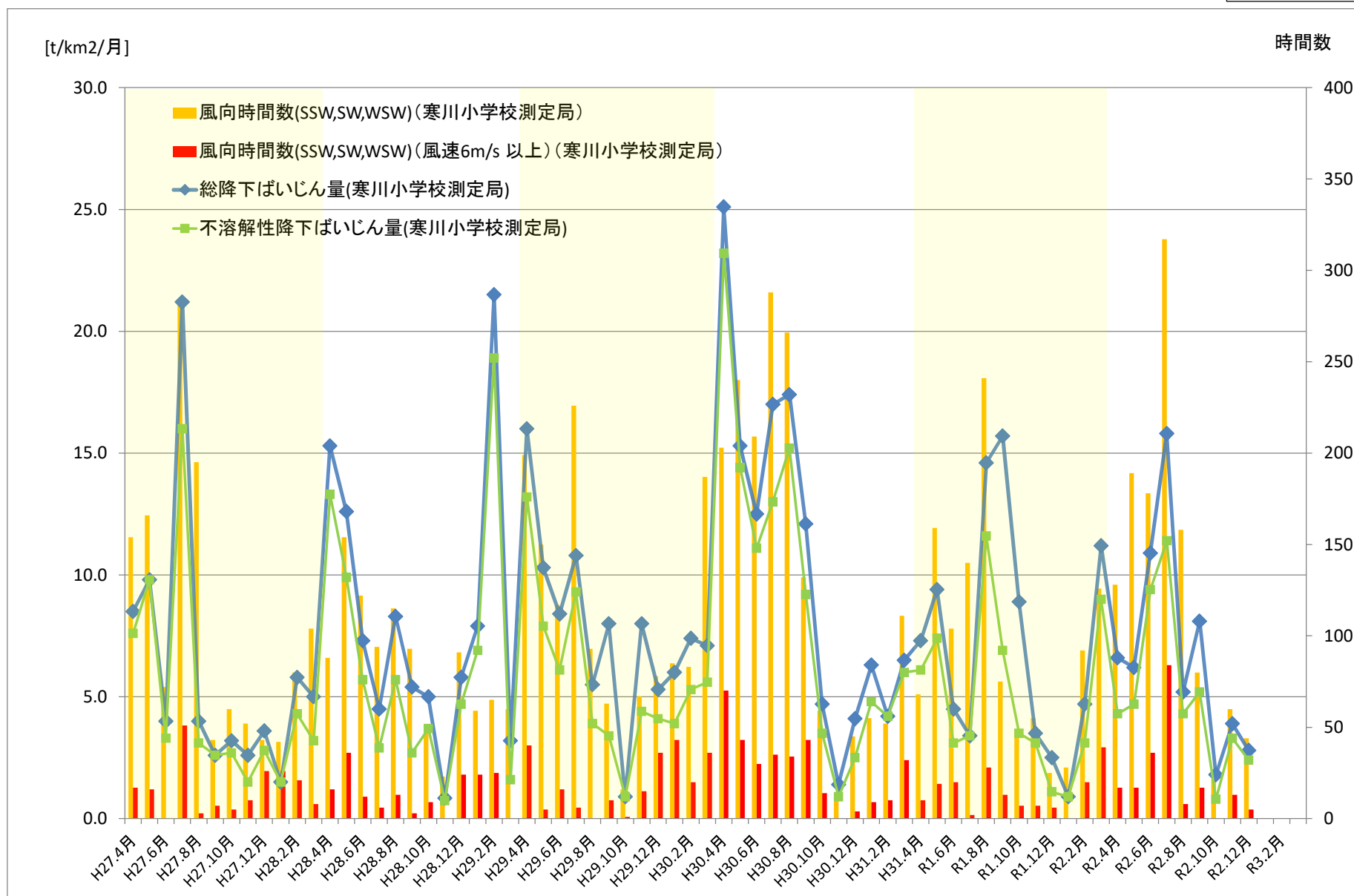
図1 寒川小学校測定局における降下ばいじん量測定結果(経月変化)
