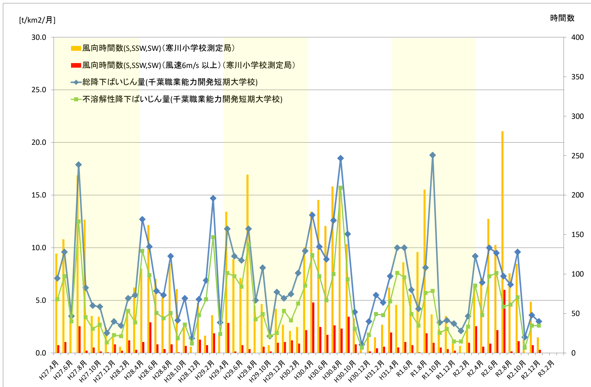
図2 千葉職業能力開発短期大学校における降下ばいじん量測定結果(経月変化)
