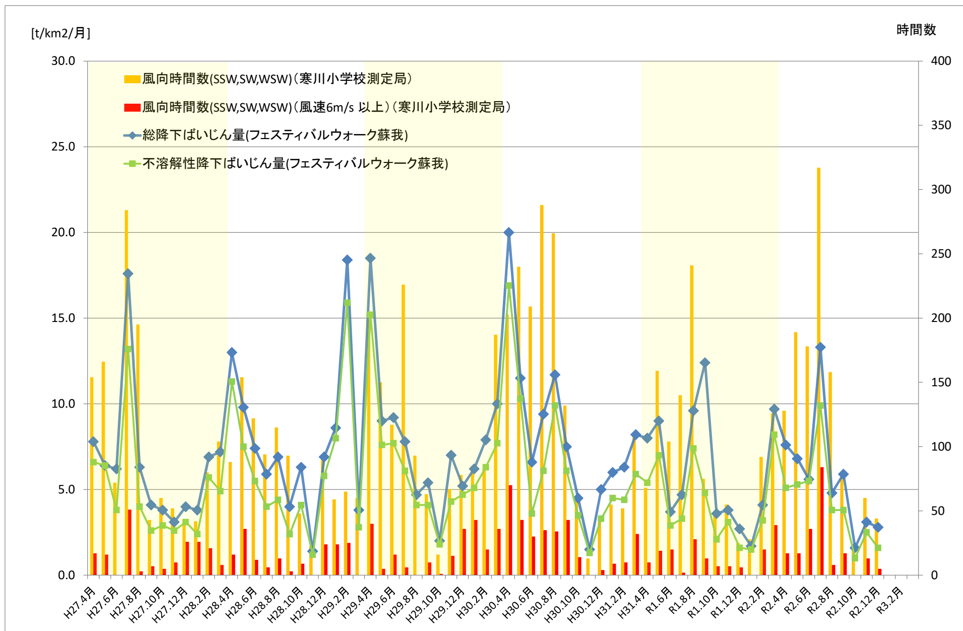
図4 フェスティバルウォーク蘇我における降下ばいじん量測定結果(経月変化)
