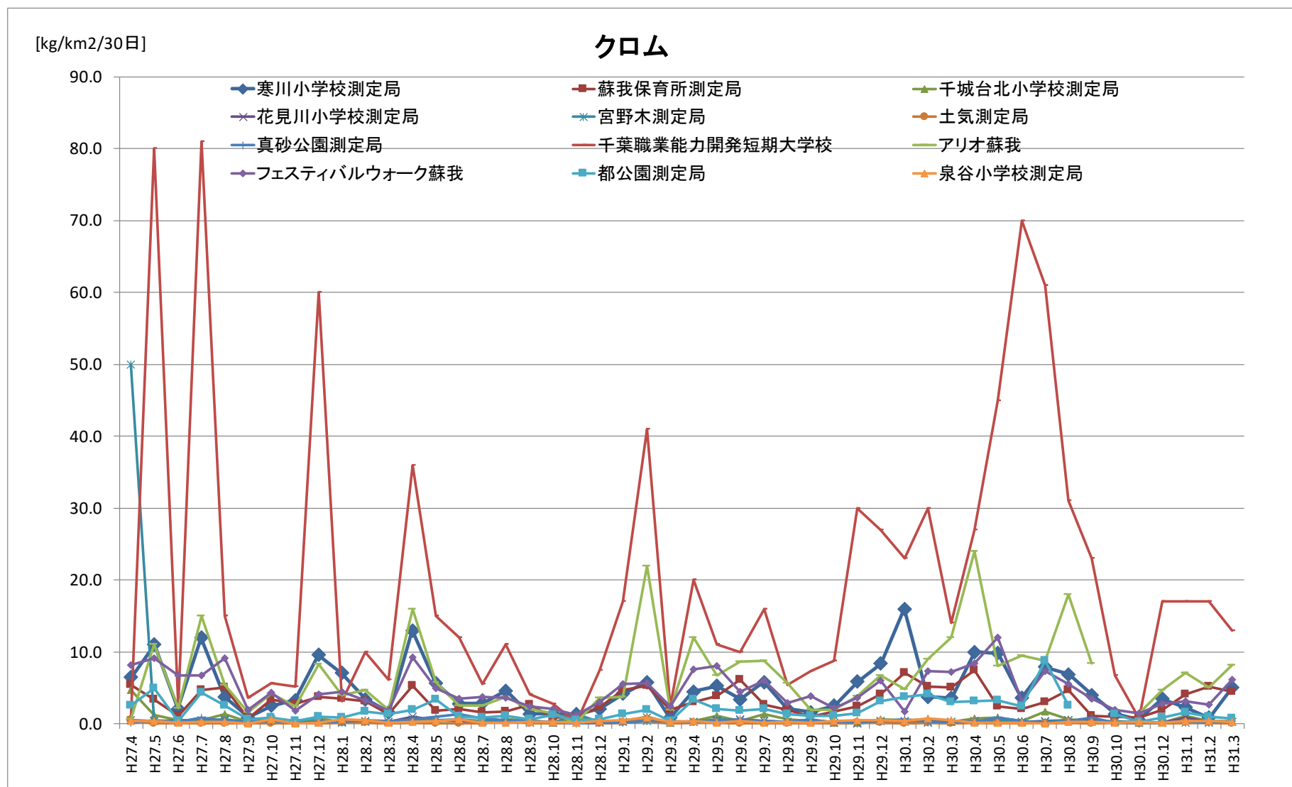
図 3.9 降下ばいじん測定結果（クロム 経月変化）
