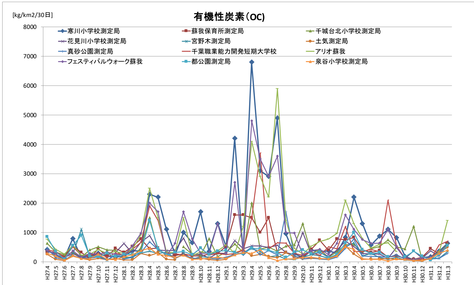
図 3.5 降下ばいじん測定結果 (有機性炭素 経月変化)
