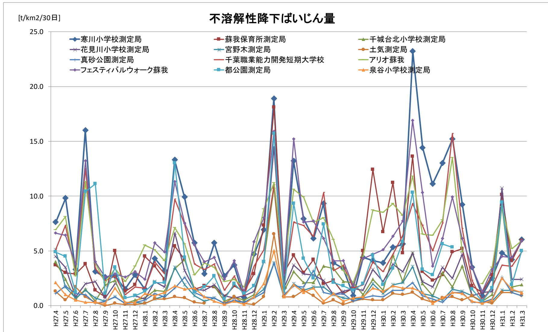
図 3.3 降下ばいじん測定結果（不溶解性降下ばいじん量 経月変化）
