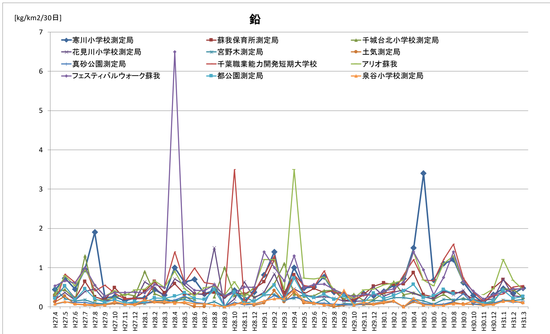
図 3.13 降下ばいじん測定結果（鉛 経月変化）
