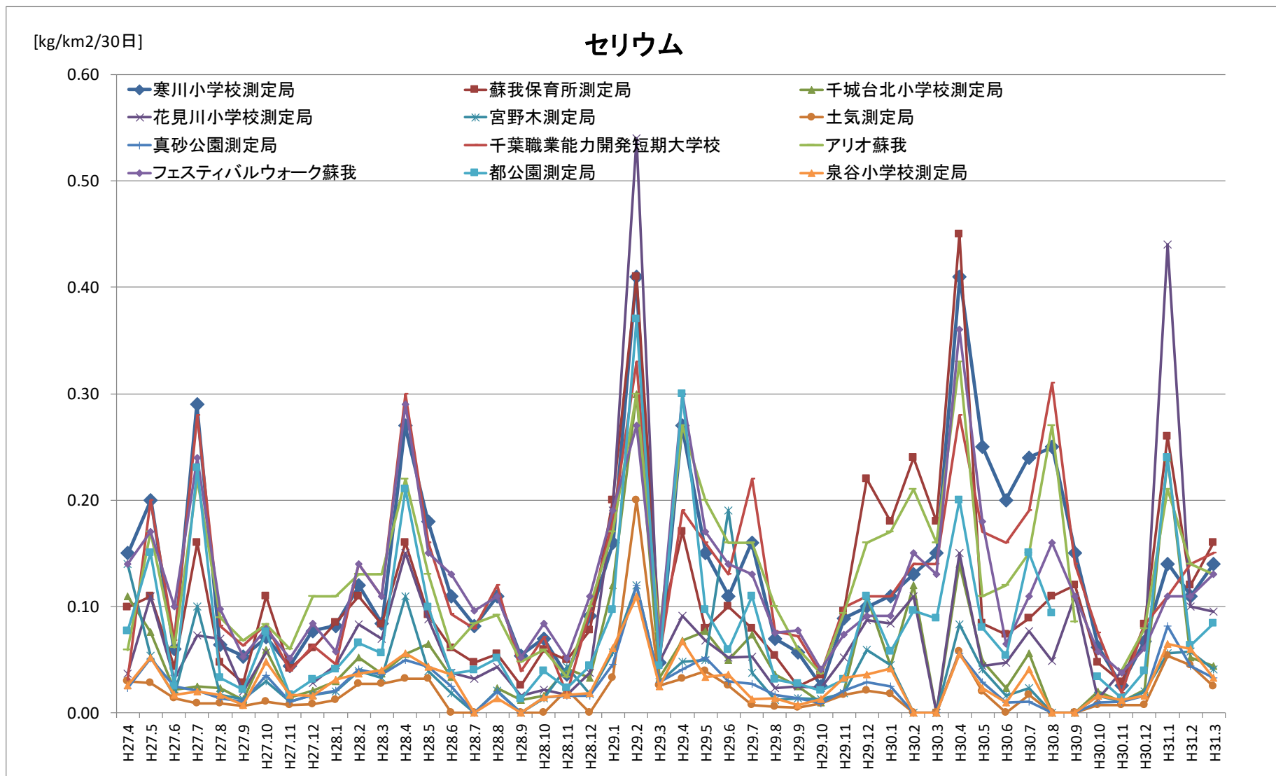
図 3.11 降下ばいじん測定結果 (セリウム 経月変化)
