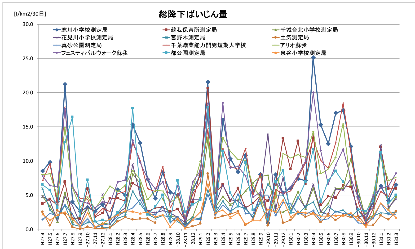
図 3.1 降下ばいじん測定結果（総降下ばいじん量 経月変化）
