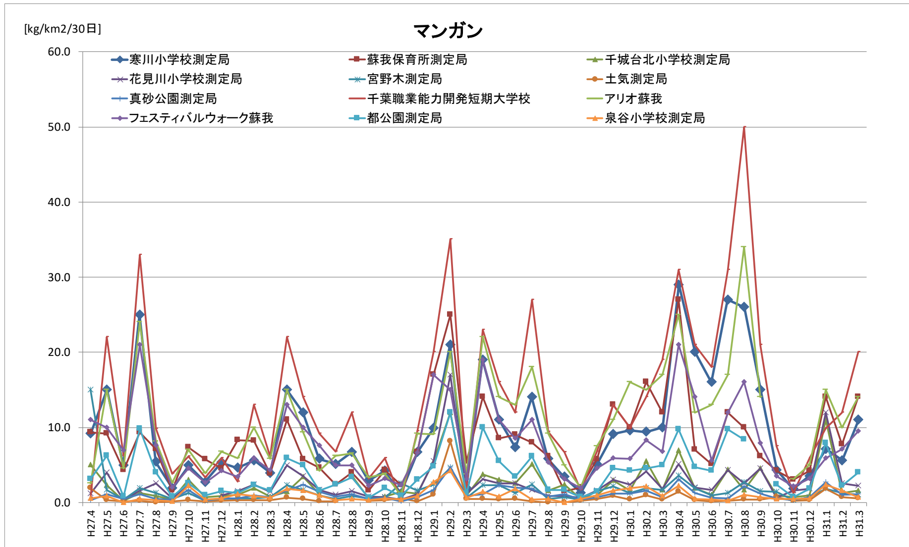
図 3.8 降下ばいじん測定結果（マンガン 経月変化）
