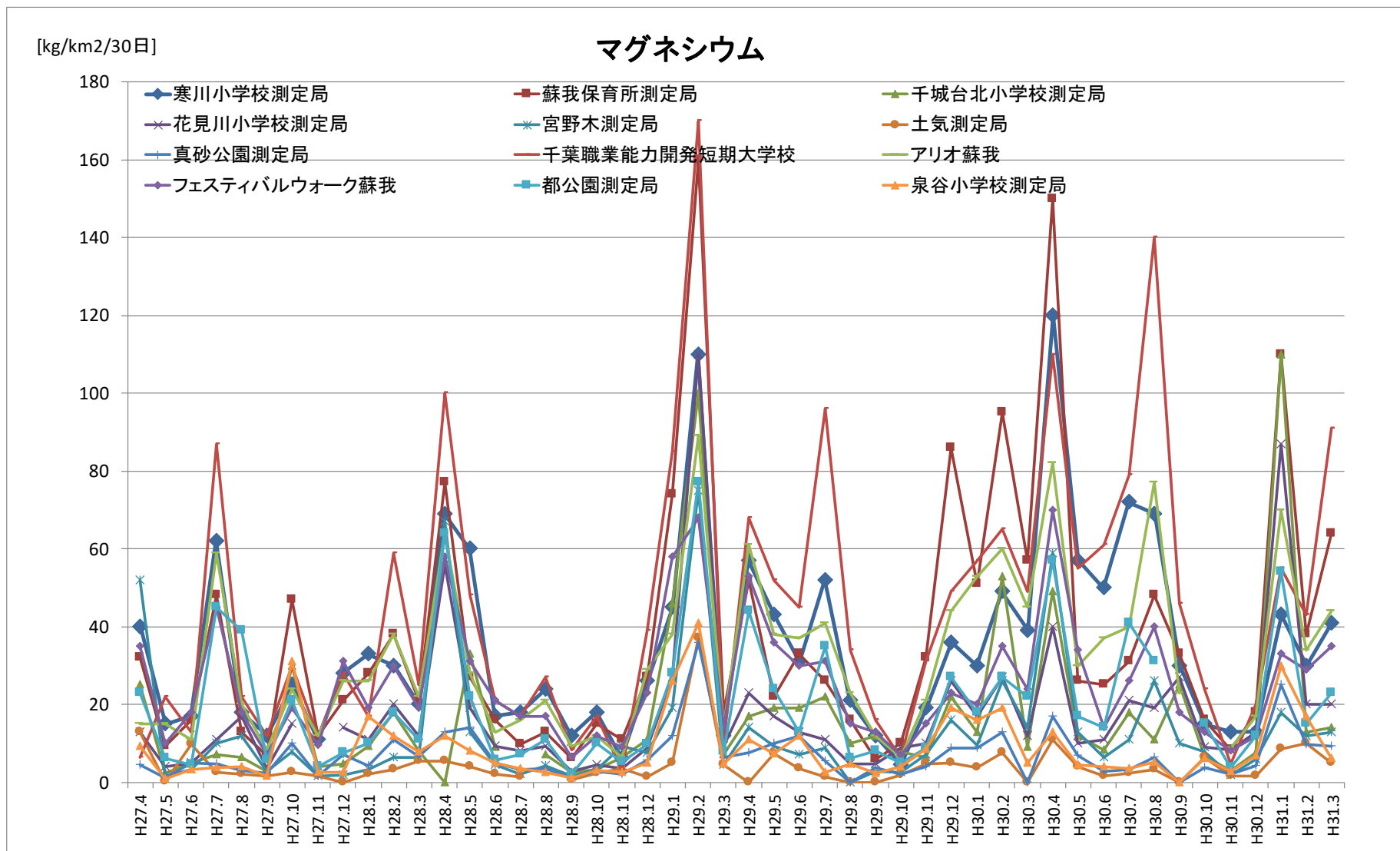
図 3.15 降下ばいじん測定結果（マグネシウム 経月変化）
