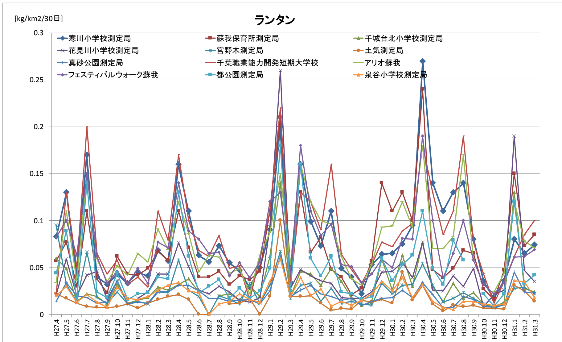
図 3.10 降下ばいじん測定結果（ランタン 経月変化）
