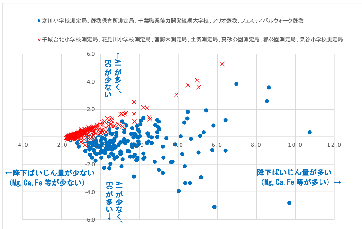
図 2.6-2(2) 主成分得点分布 (主成分 1×主成分 2)
