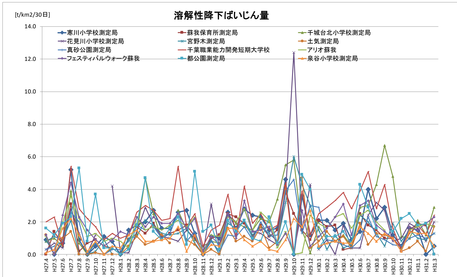
図 3.2 降下ばいじん測定結果（溶解性降下ばいじん量 経月変化）
