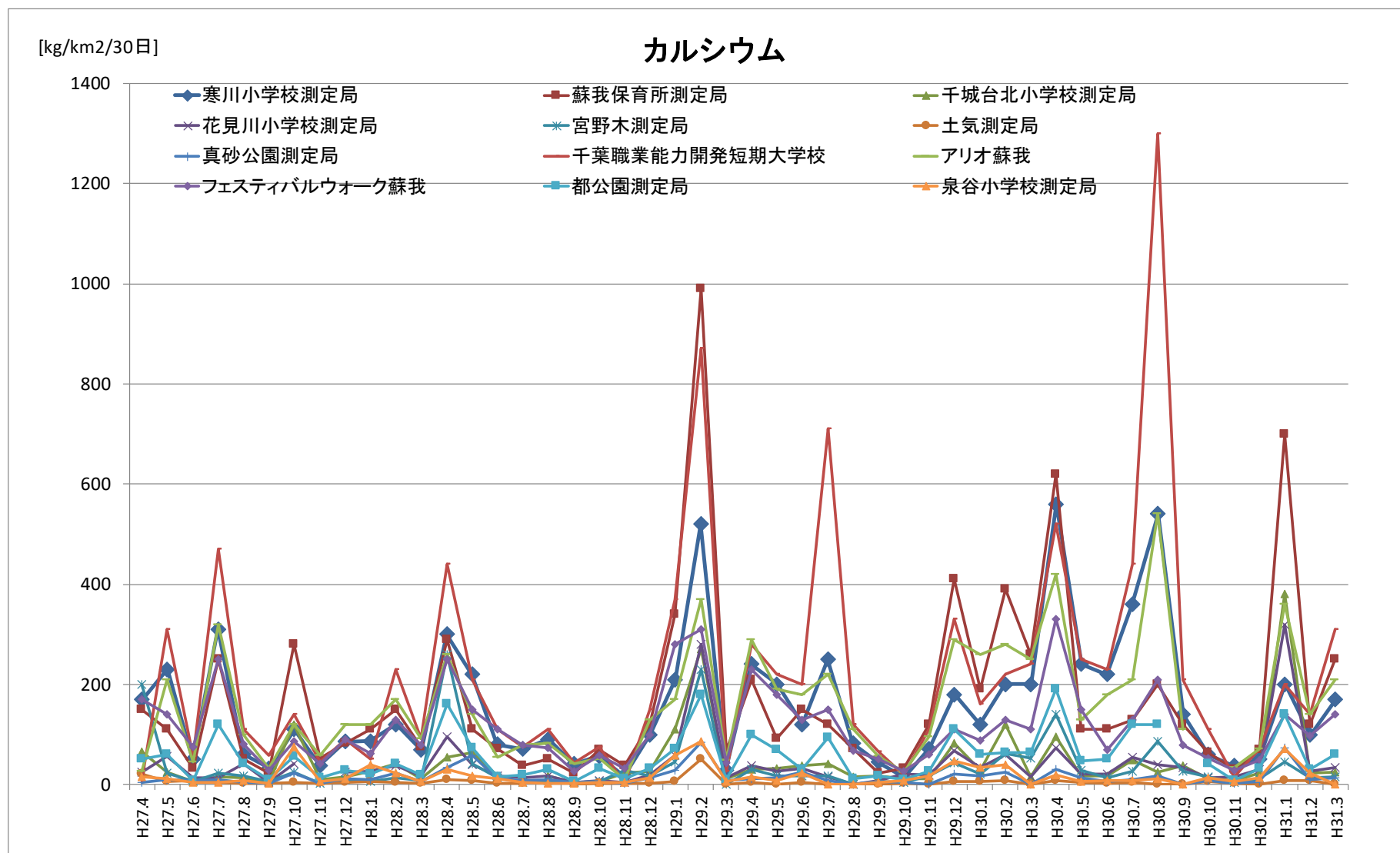
図 3.7 降下ばいじん測定結果（カルシウム 経月変化）
