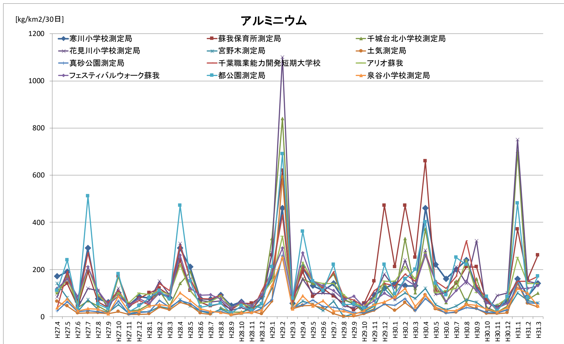
図 3.12 降下ばいじん測定結果（アルミニウム 経月変化）
