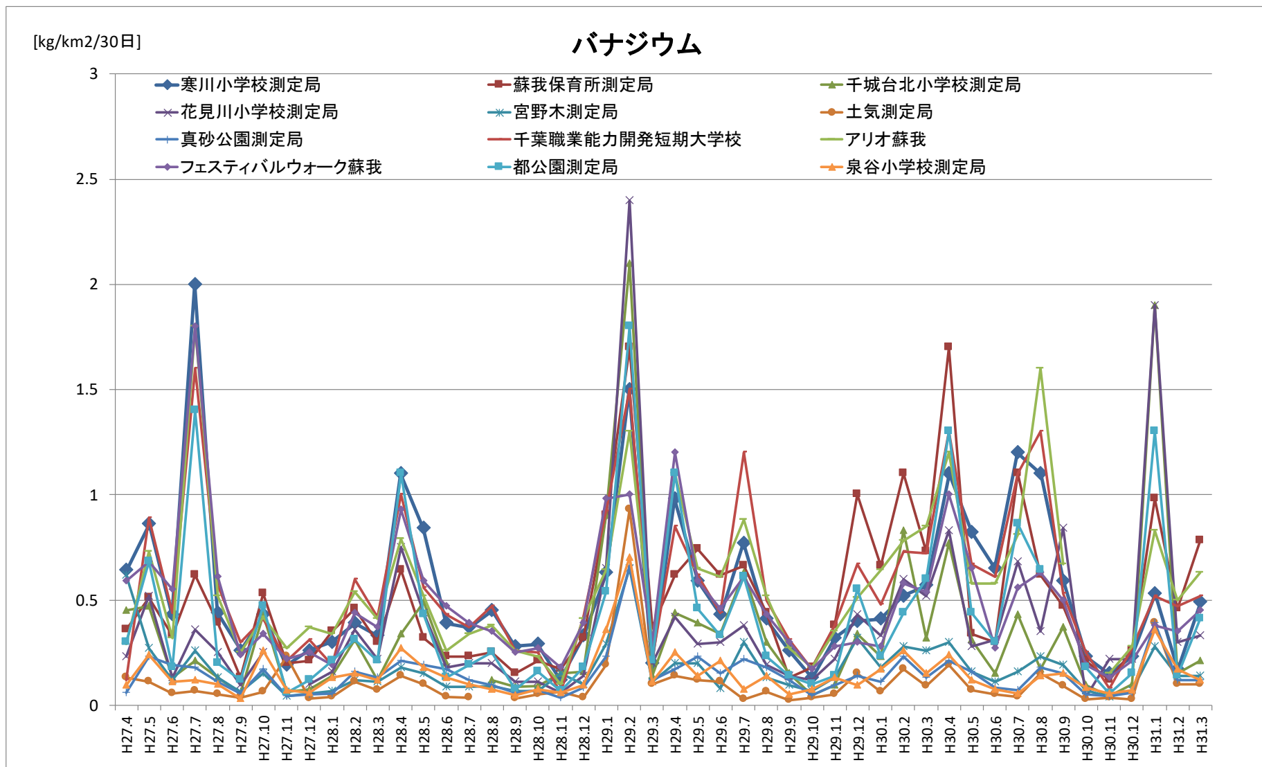
図 3. 14 降下ばいじん測定結果 (バナジウム 経月変化)
