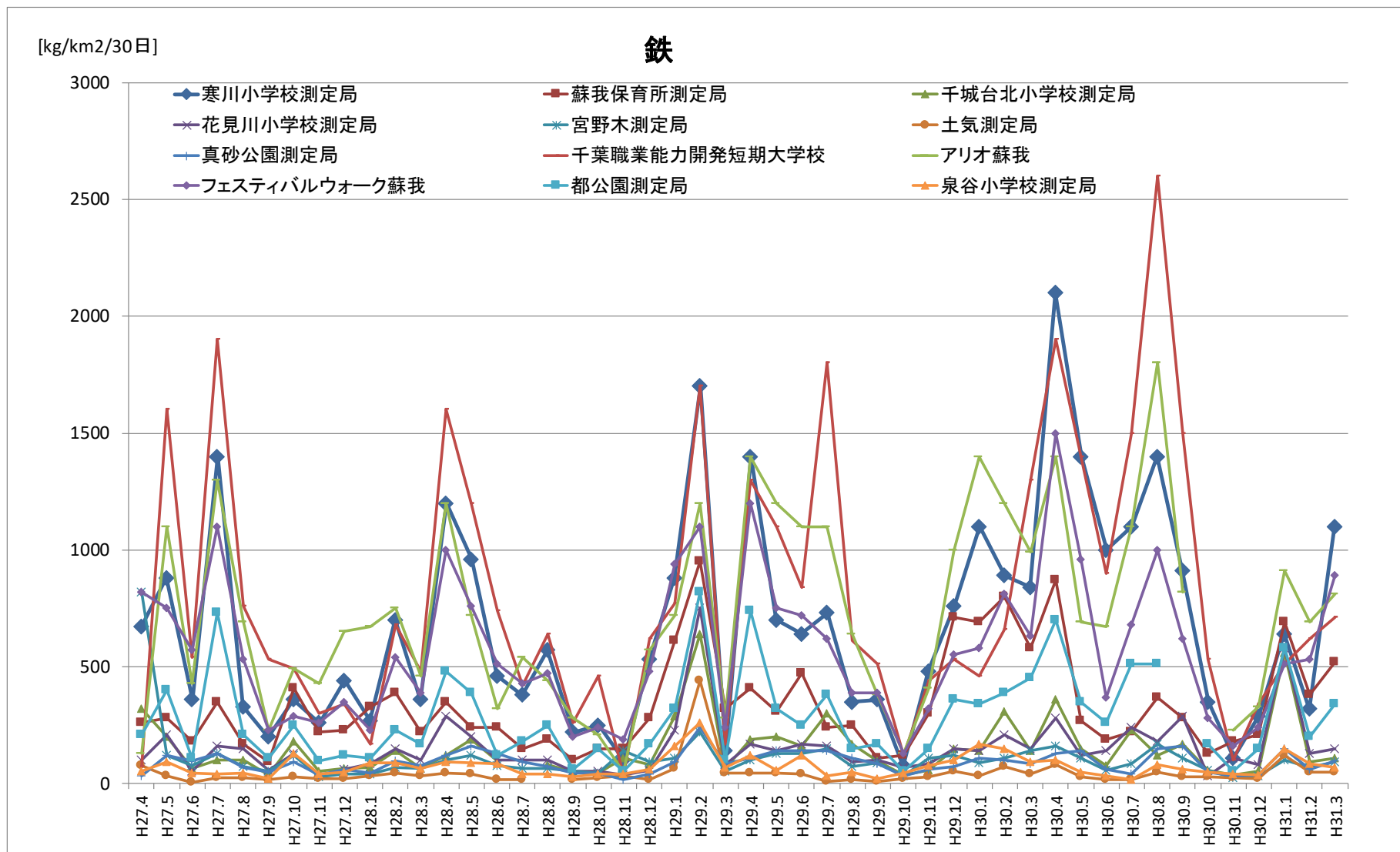
図 3.6 降下ばいじん測定結果（鉄 経月変化）
