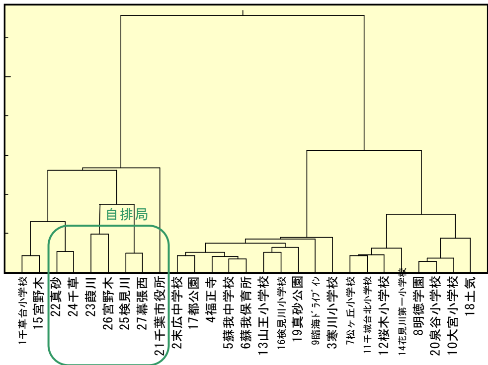
図 2(2) 樹形図 (平成 19 年度、日平均値、二酸化窒素)
