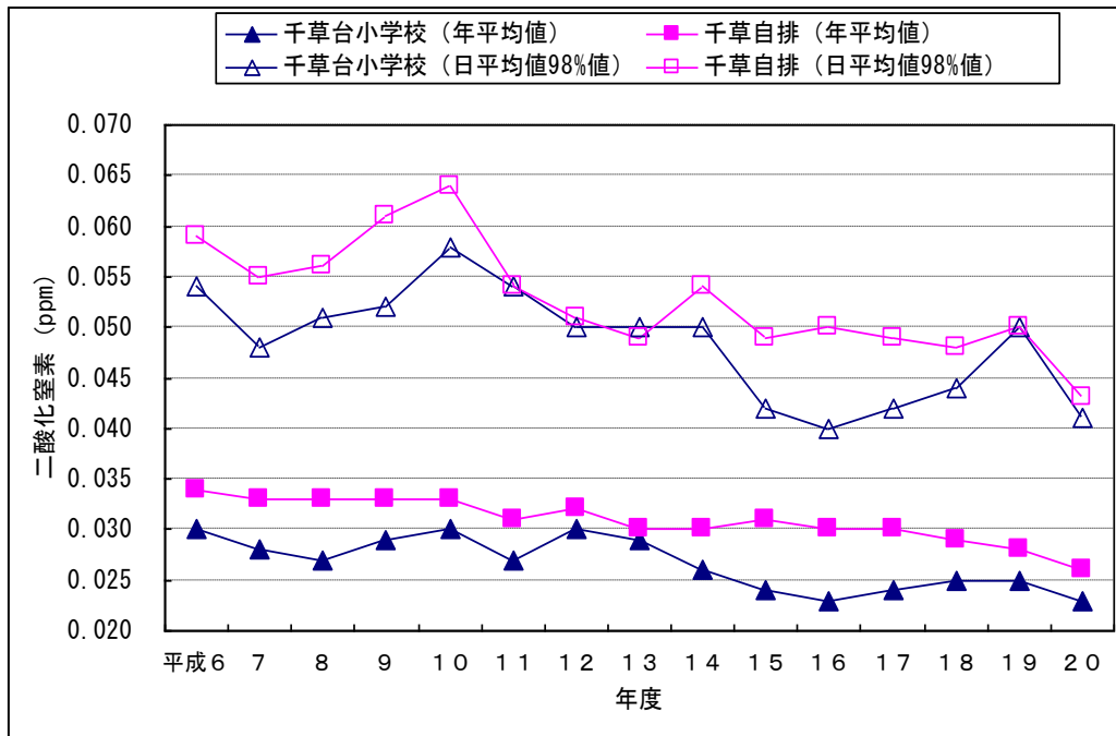
図3 二酸化窒素濃度の経年変化（年平均值、日平均値98%値）
