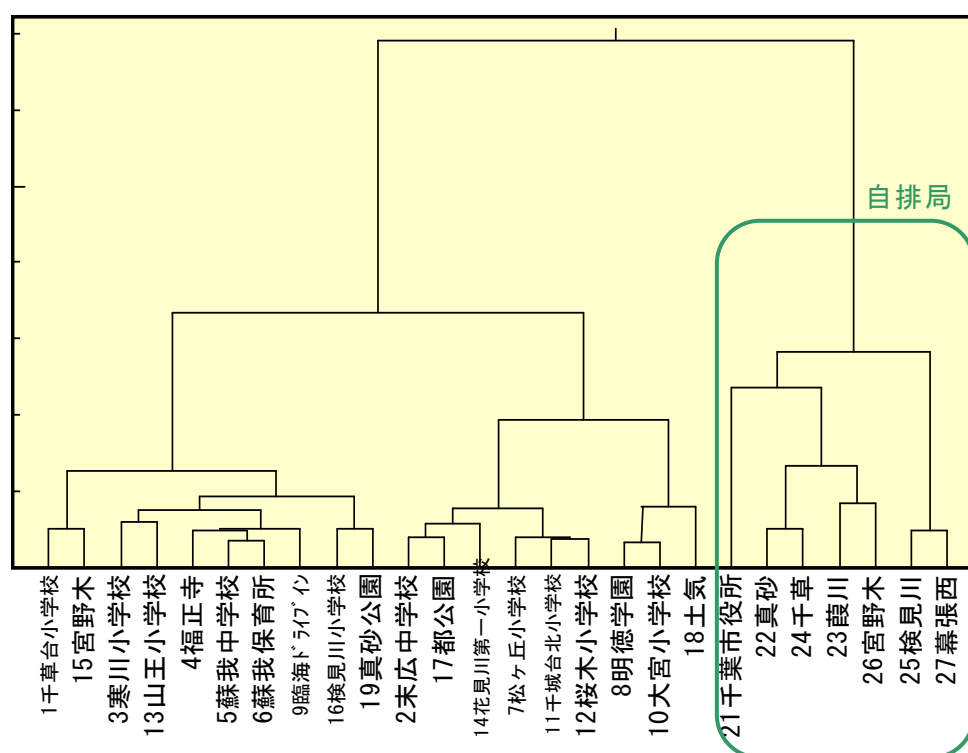
図 2(1) 樹形図（平成 18 年度、日平均値、二酸化窒素）
