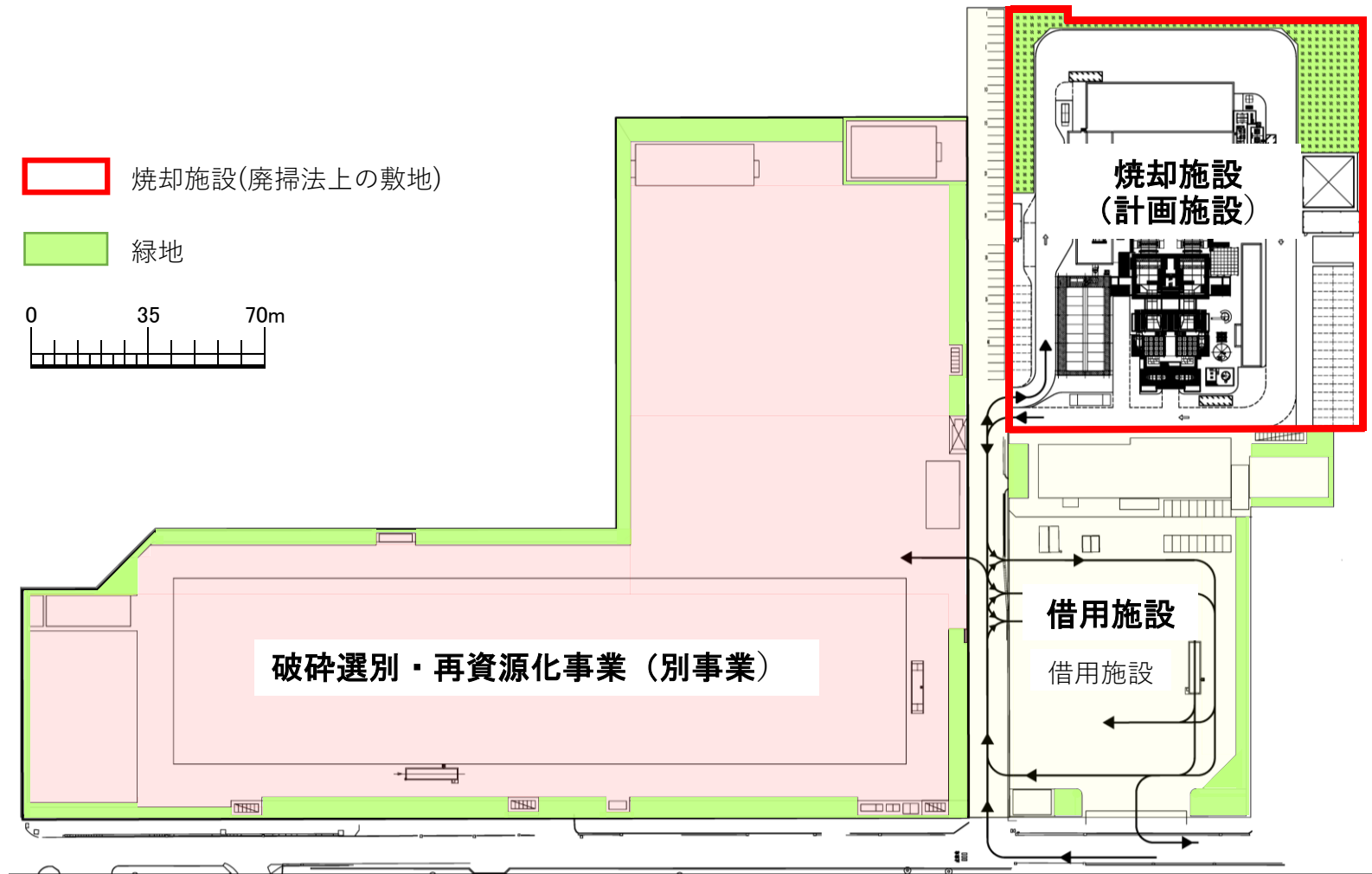
別事業(破砕選別・再資源化事業)・借用施設を含む全体配置計画
