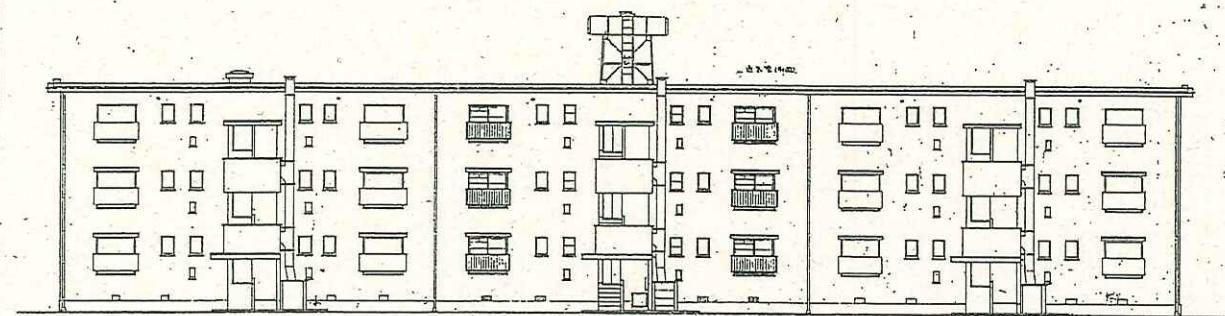
北立面 图 1:100
