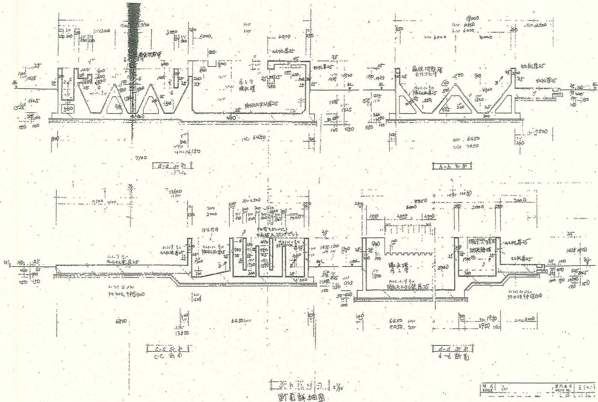
污水管断面详细图
