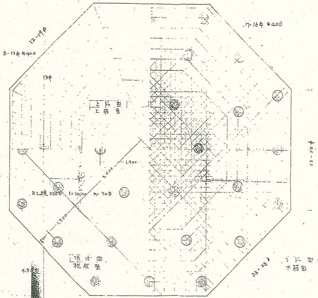
煙突基礎配筋圖
