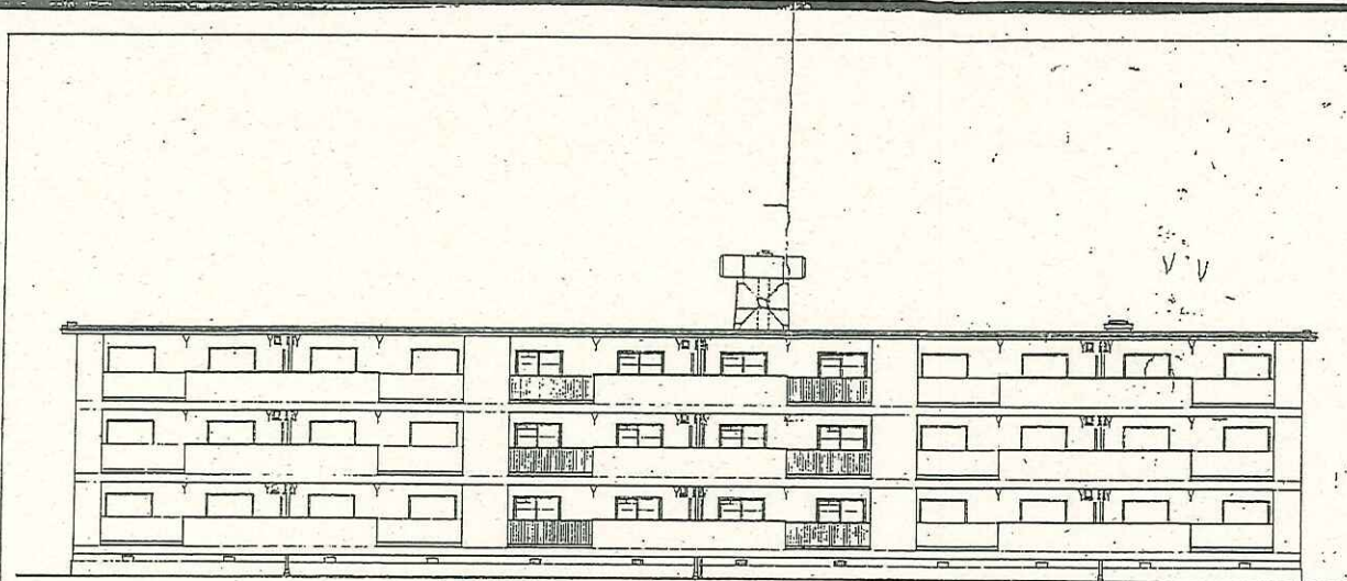
东立面 图 1:100
