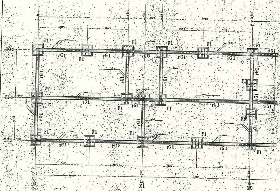
基礎配筋詳細図 SCALE 1/50
