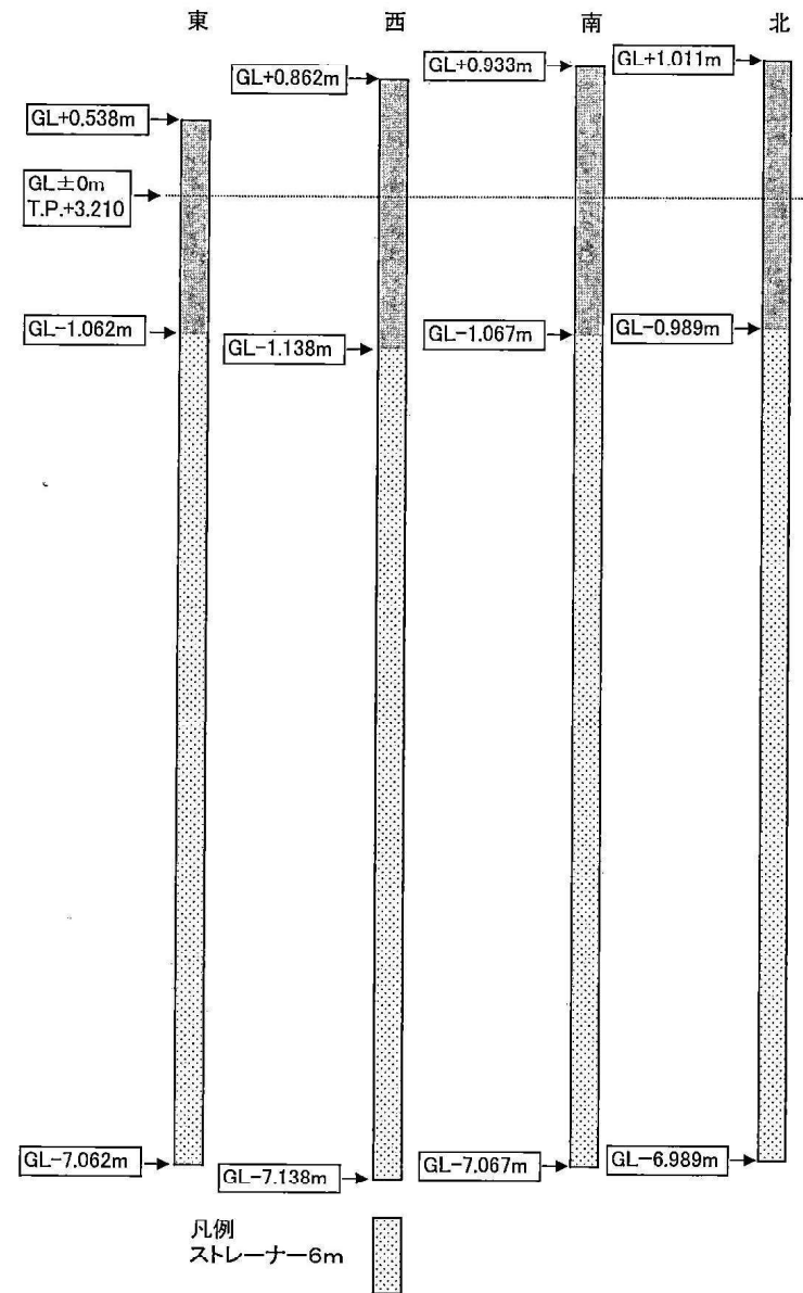
旧新港清掃工場観測井設置深度概念図
