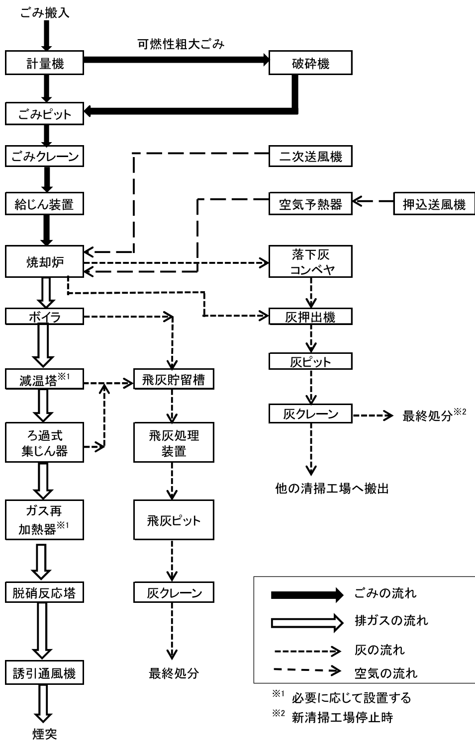
図1 ごみ処理基本フロー
