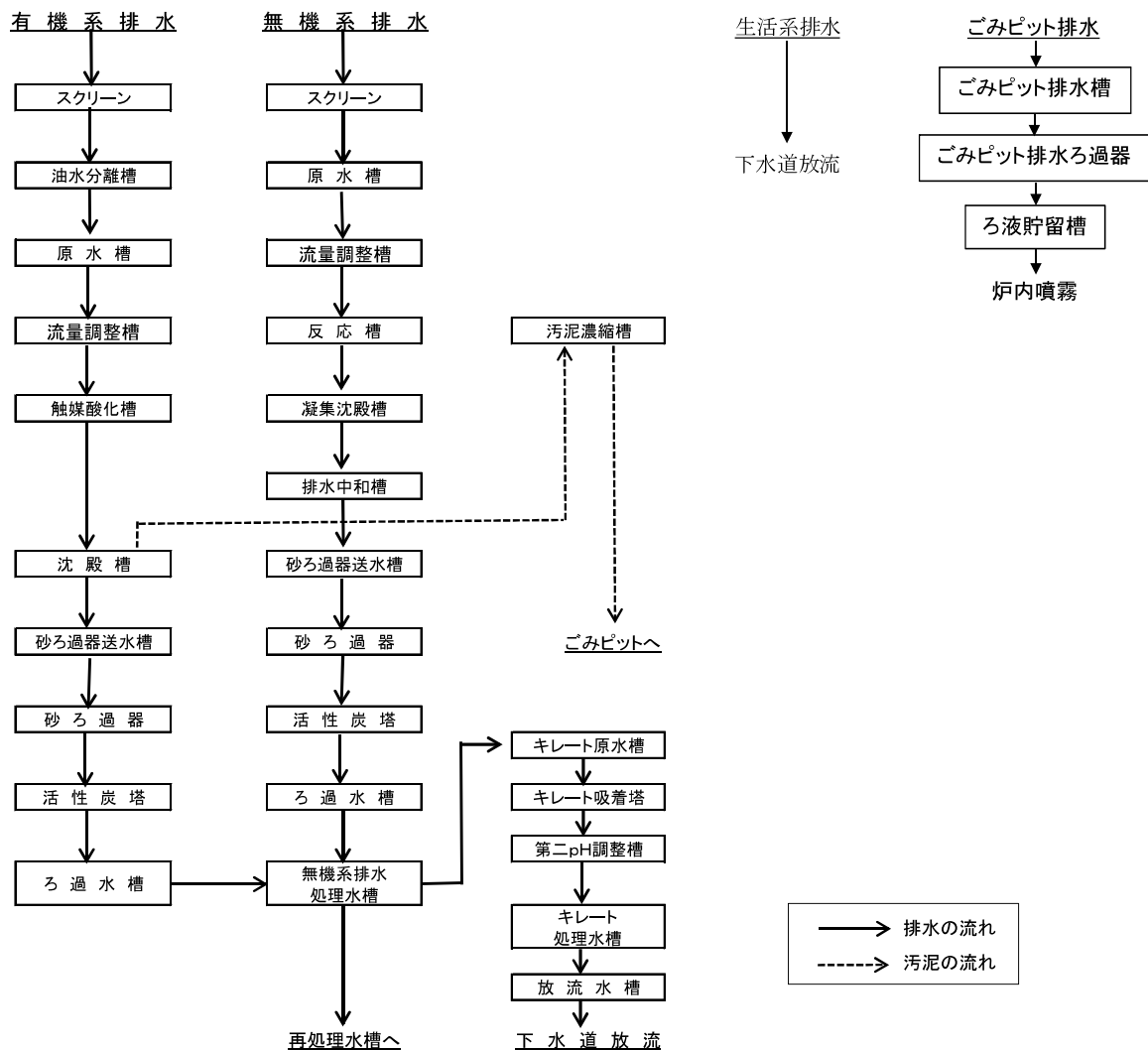
図4 排水処理基本フロー
