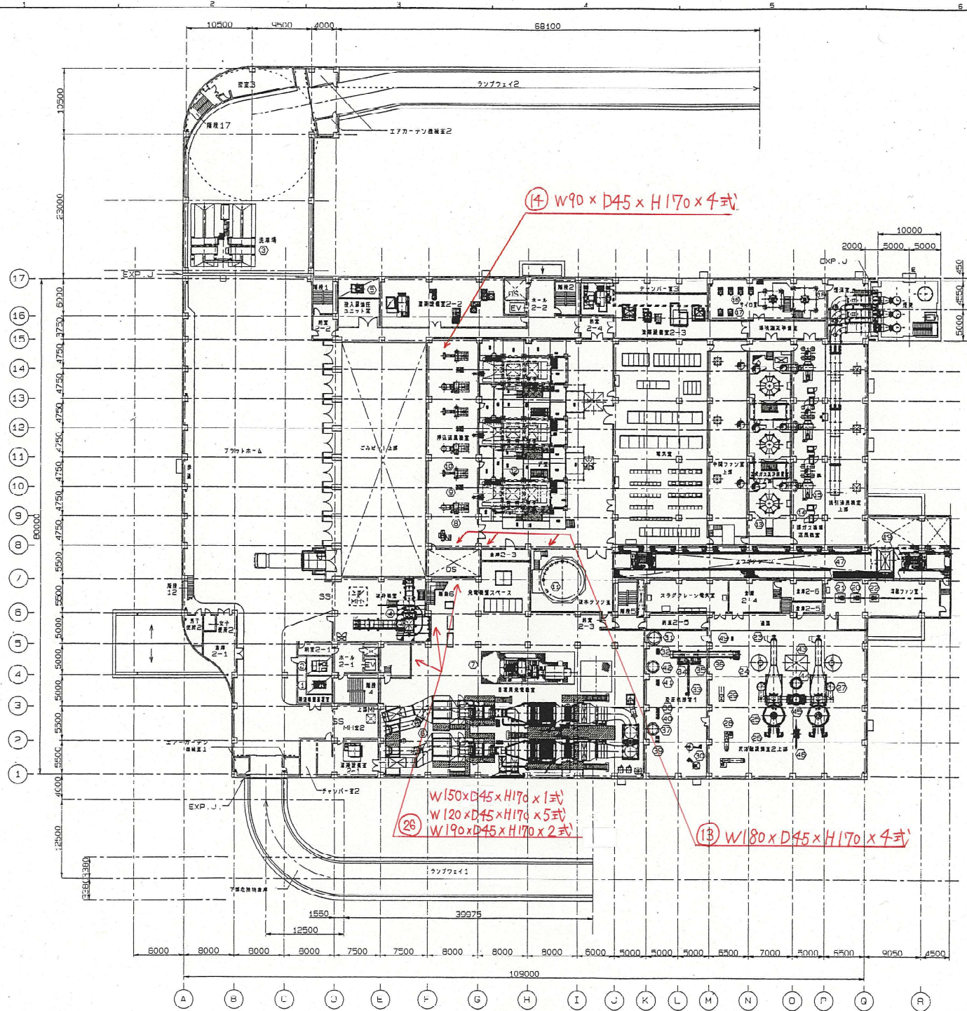
中2階平面図 注: 特記なき限り、床レベルは 1FL+6, 500 とする。
