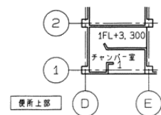
便所上部
