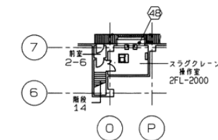
中2階平面図
