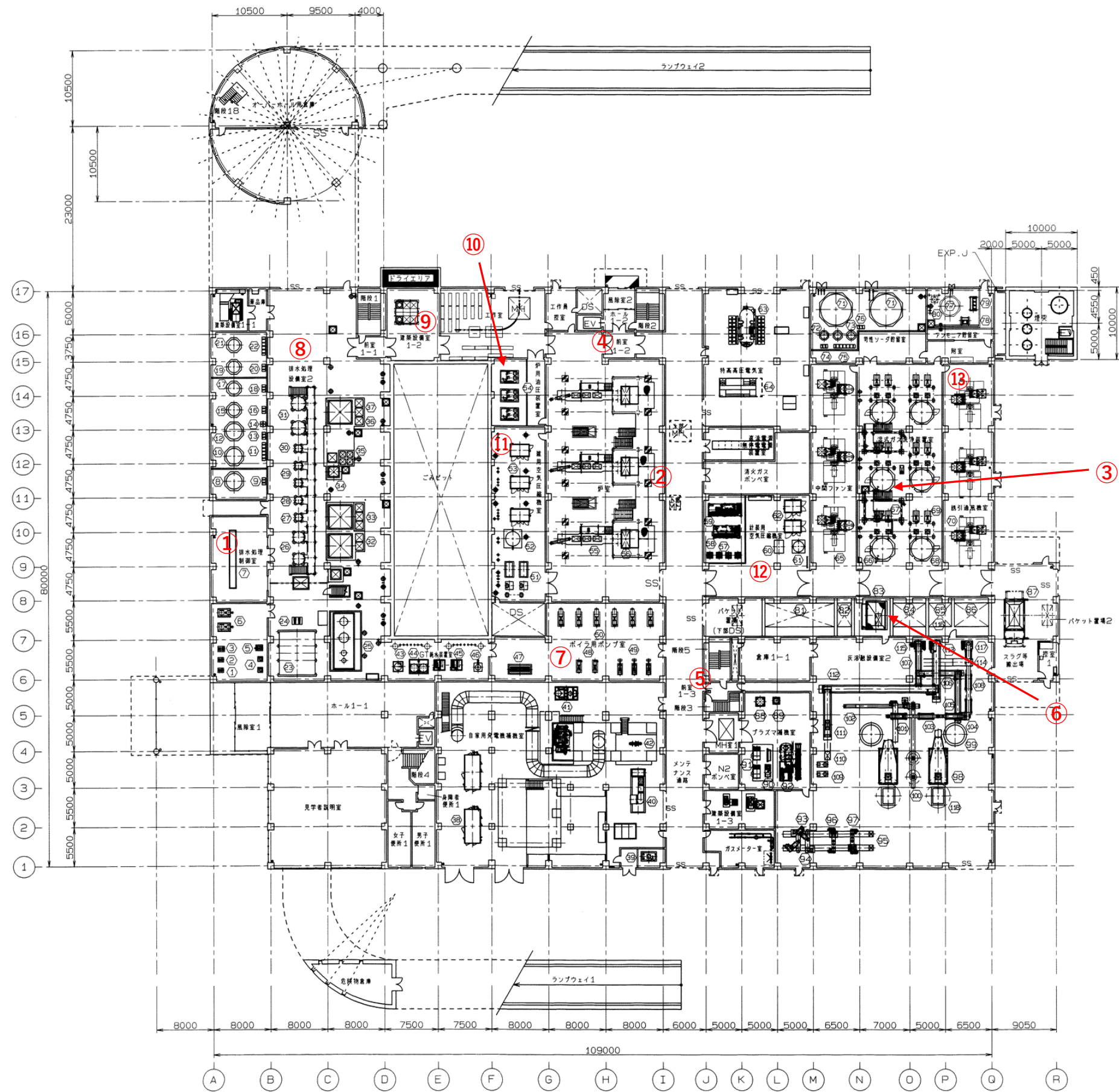
1階平面図
