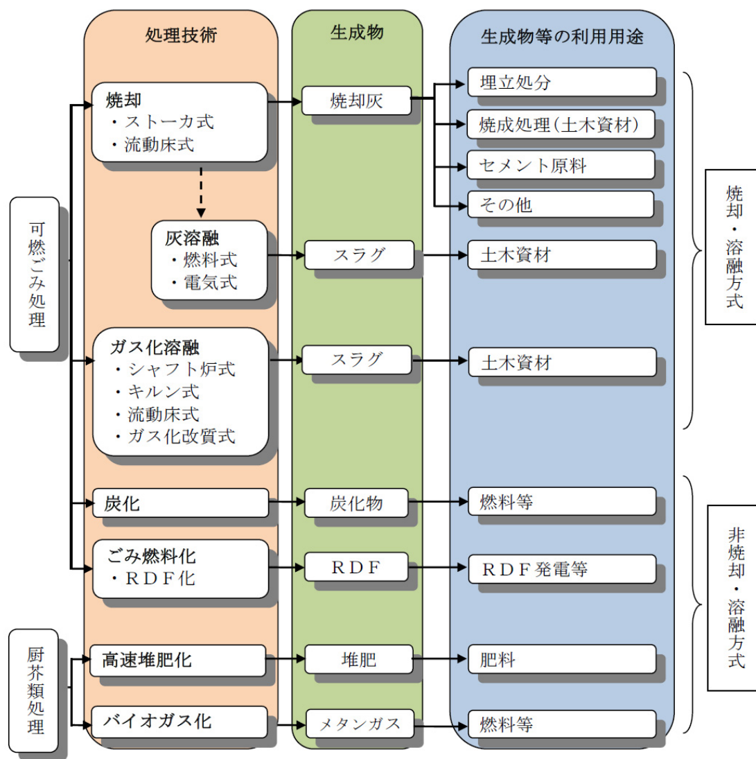
図2-5 主要な可燃ごみ処理技術
