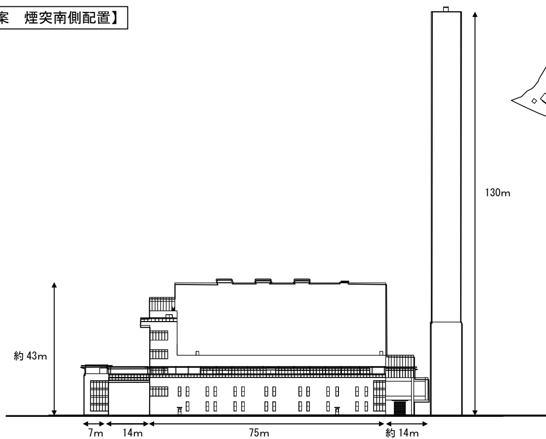
北側立面図
