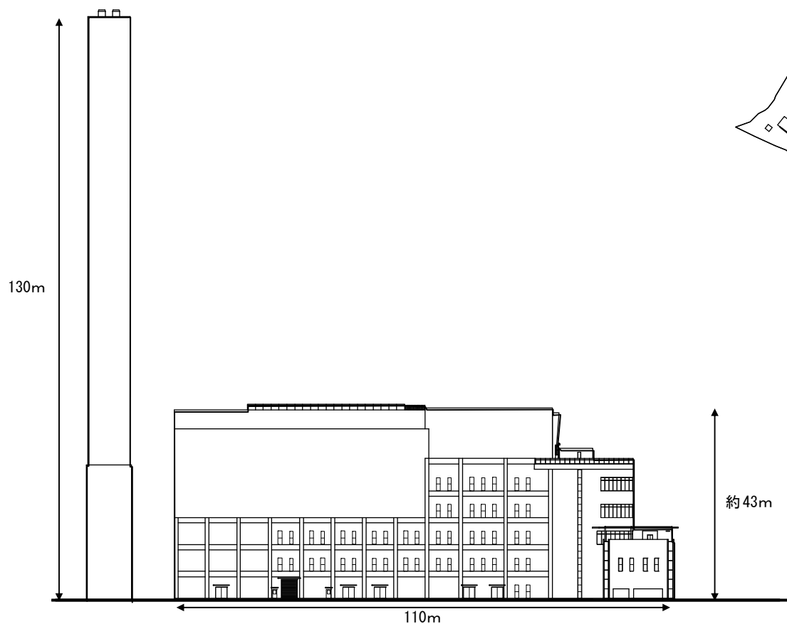
東側立面図
