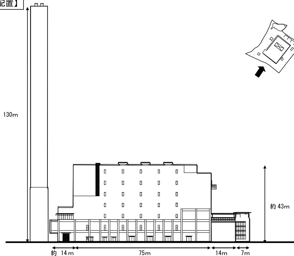
南側立面図
