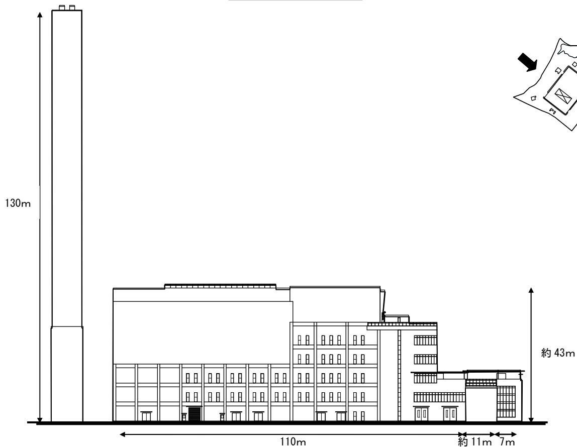
図 2-7 (2) 建築計画 (立面図)
