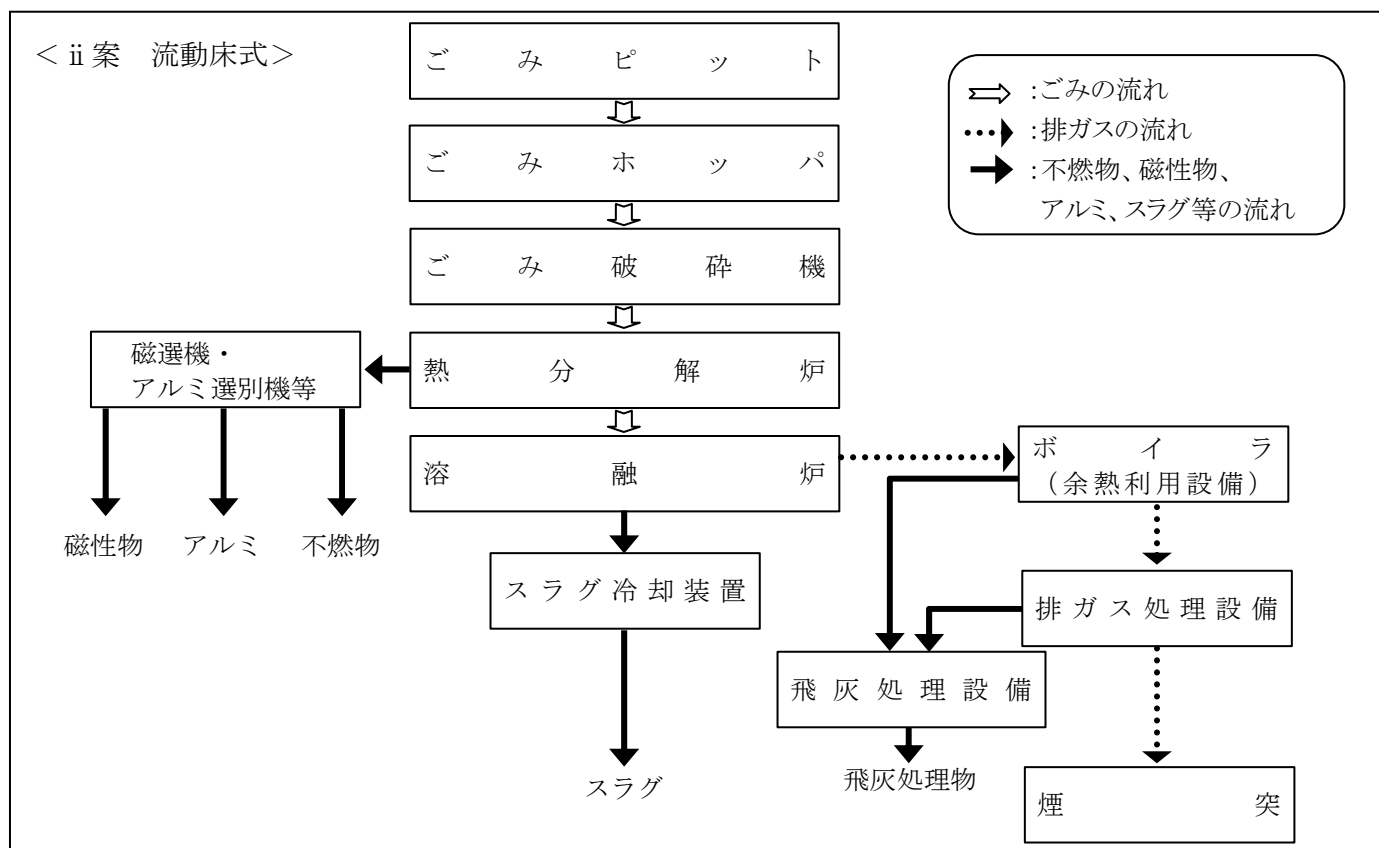
図2-10 流動床式の基本フロー
