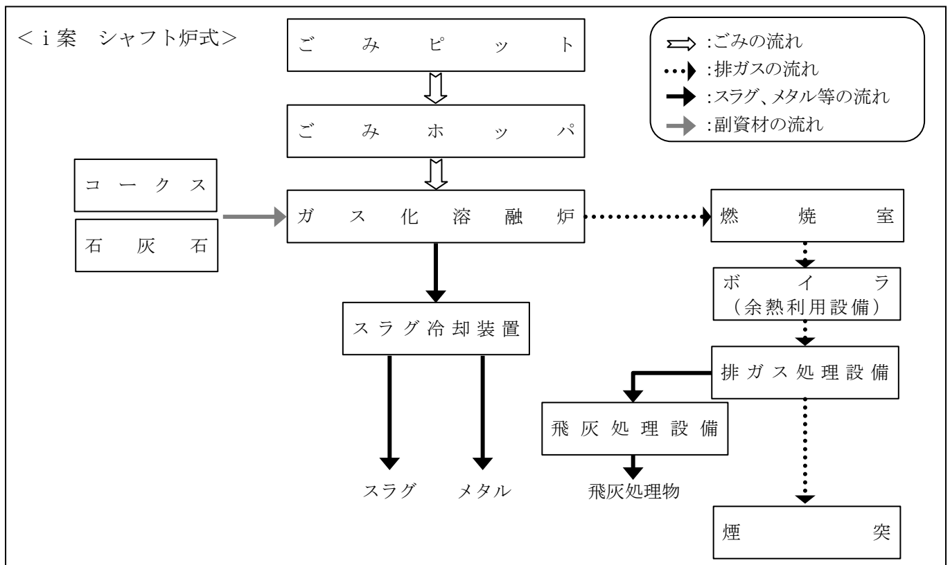
図2-9 シャフト炉式の基本フロー
