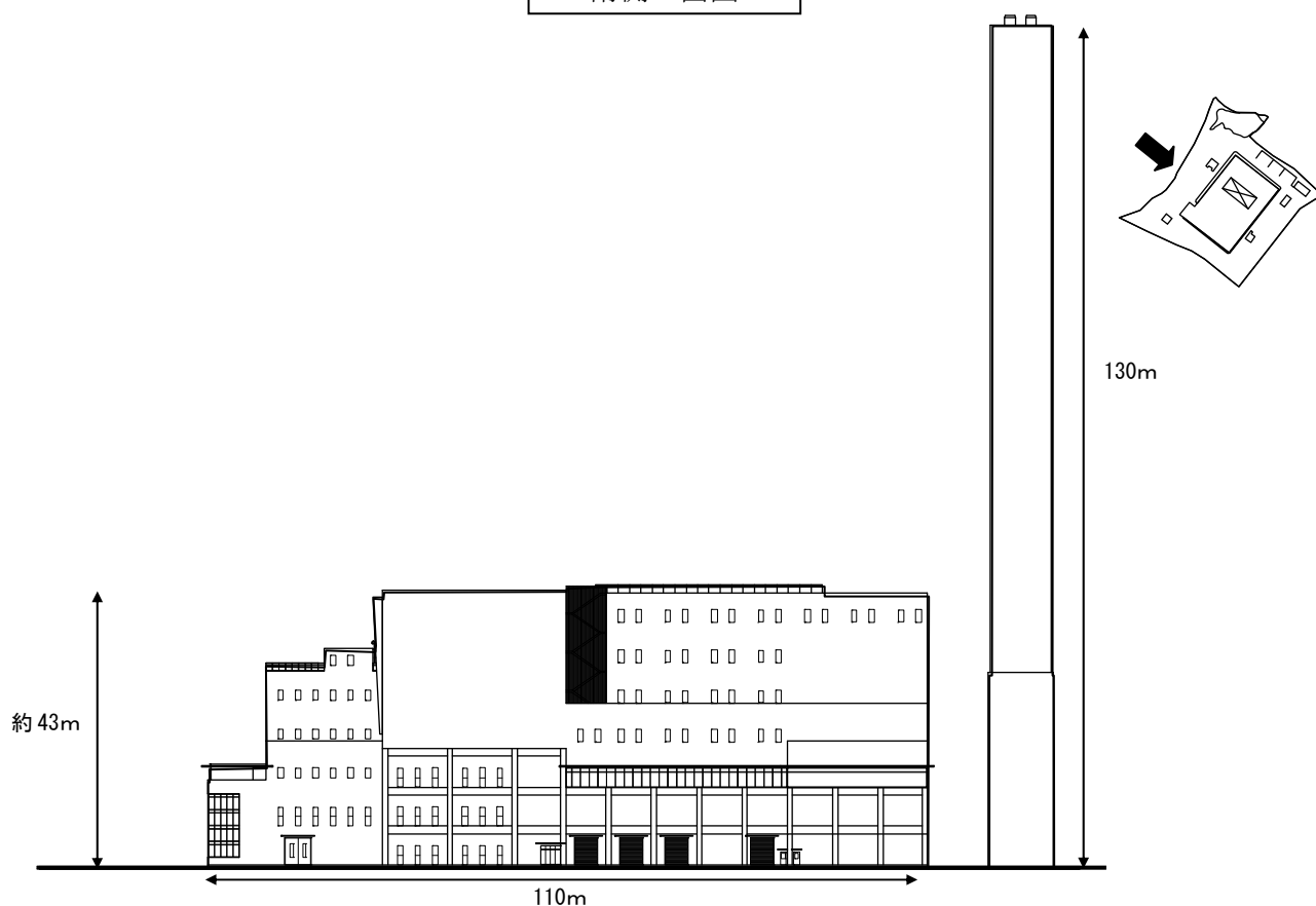
西側立面図
