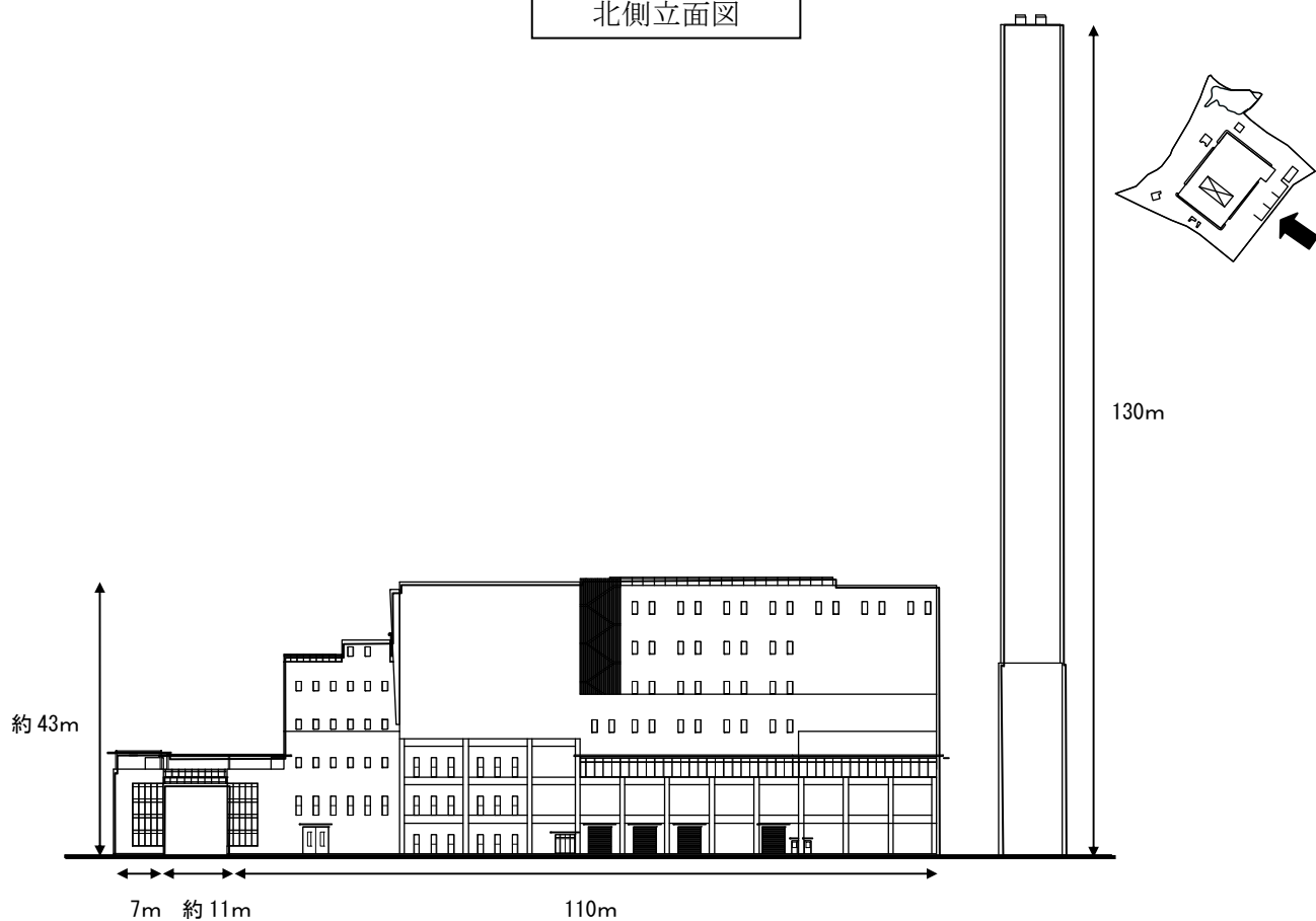
東側立面図
