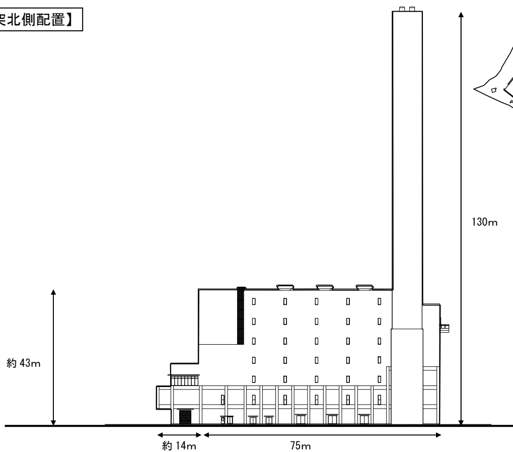
北側立面図
