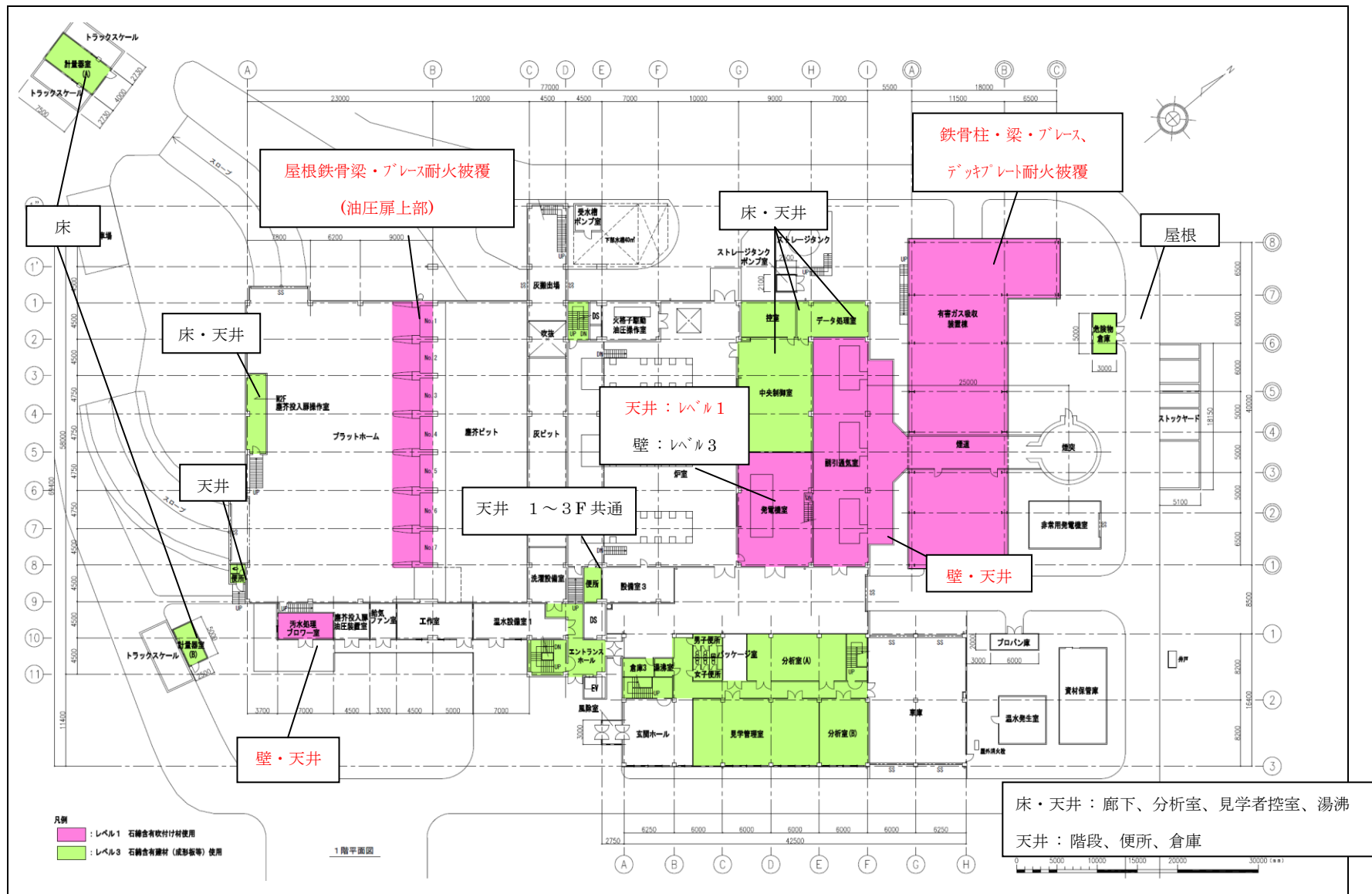
石綿混入物位置図（工場棟・管理棟 1階平面図 配置図）
