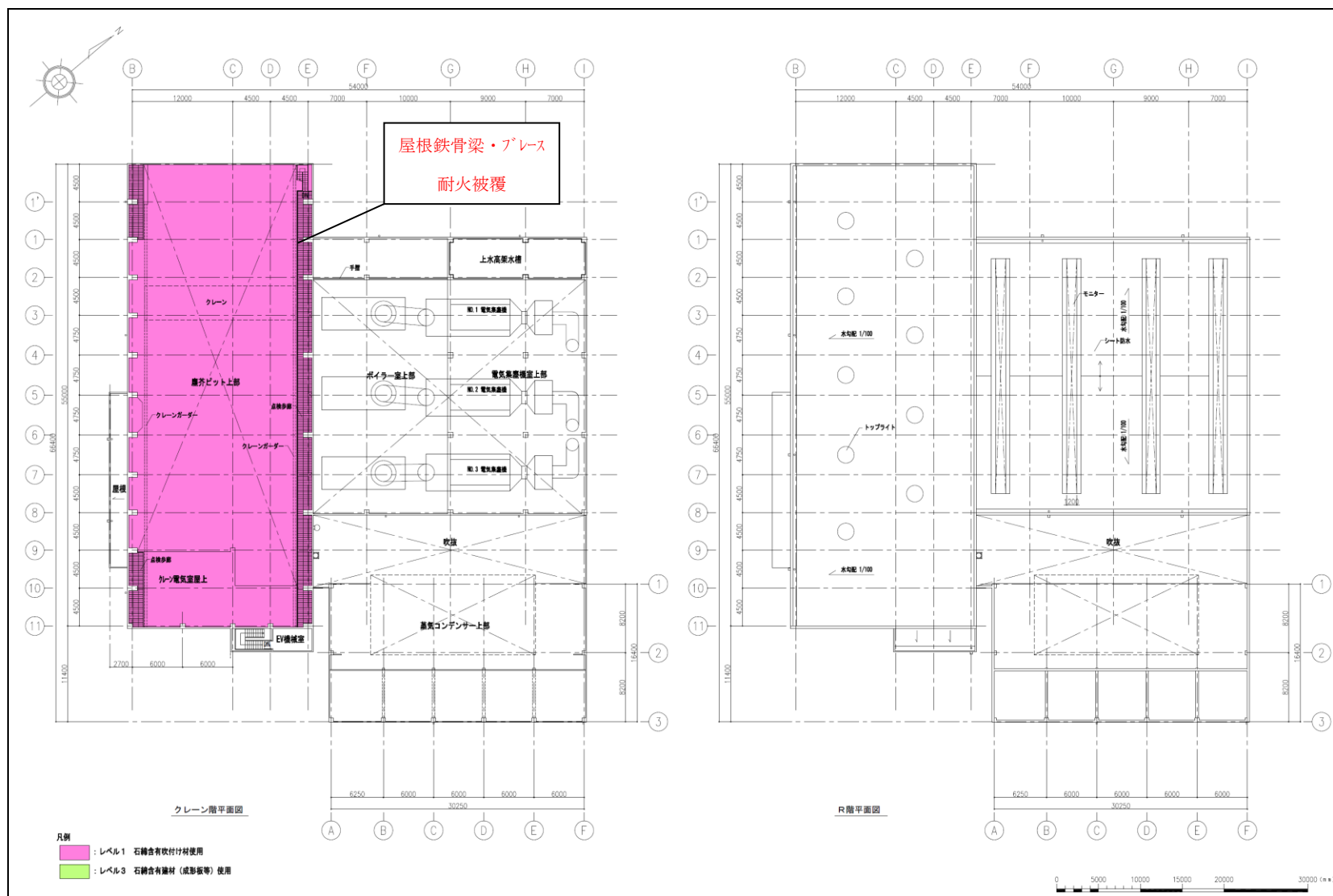
石綿混入物位置図（工場棟 クレーン階、屋上階平面図）
