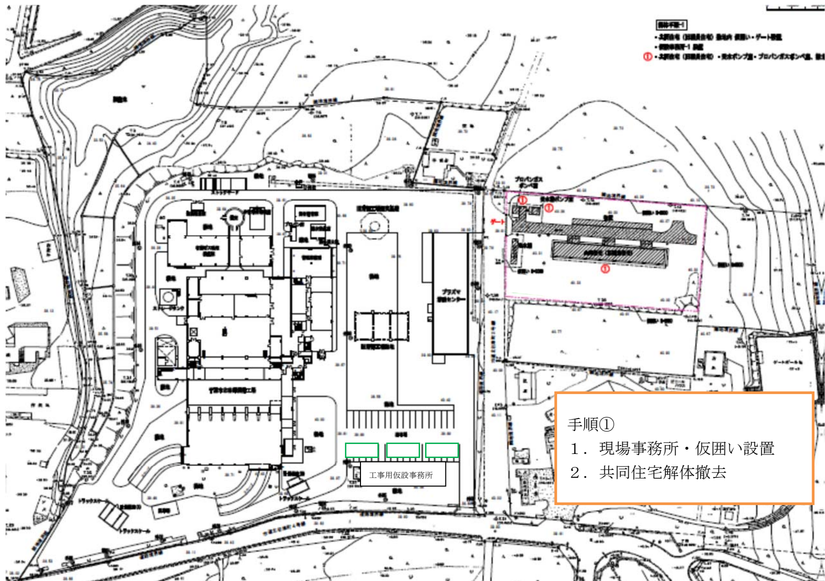
解体工事手順①
