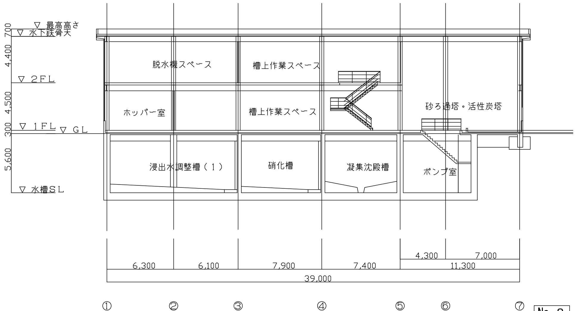
A-A断面図 S=1/150
