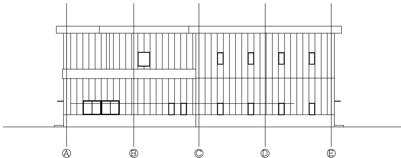
北側立面図 S=1/150
