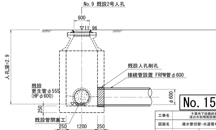
導水管切替詳細断面図
