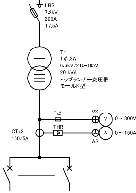
低圧電灯盤 1φ,3W,200-100V
