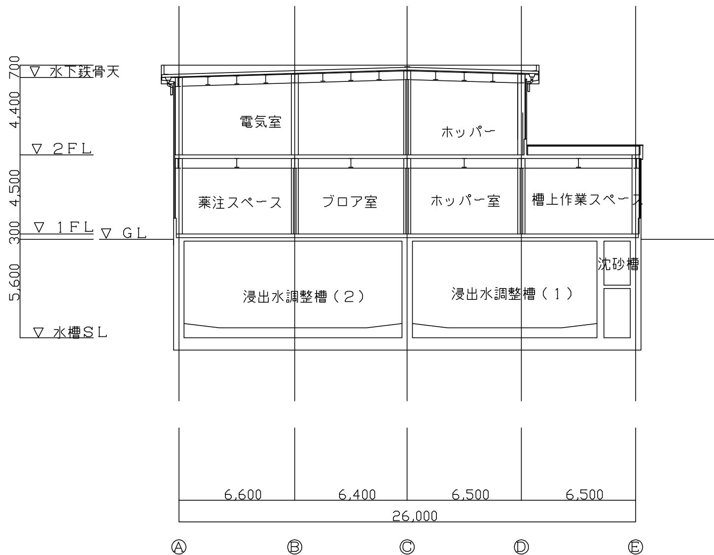
C-C断面図 S=1/150
