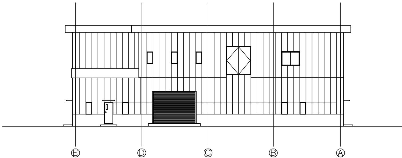
南側立面図 S=1/150
