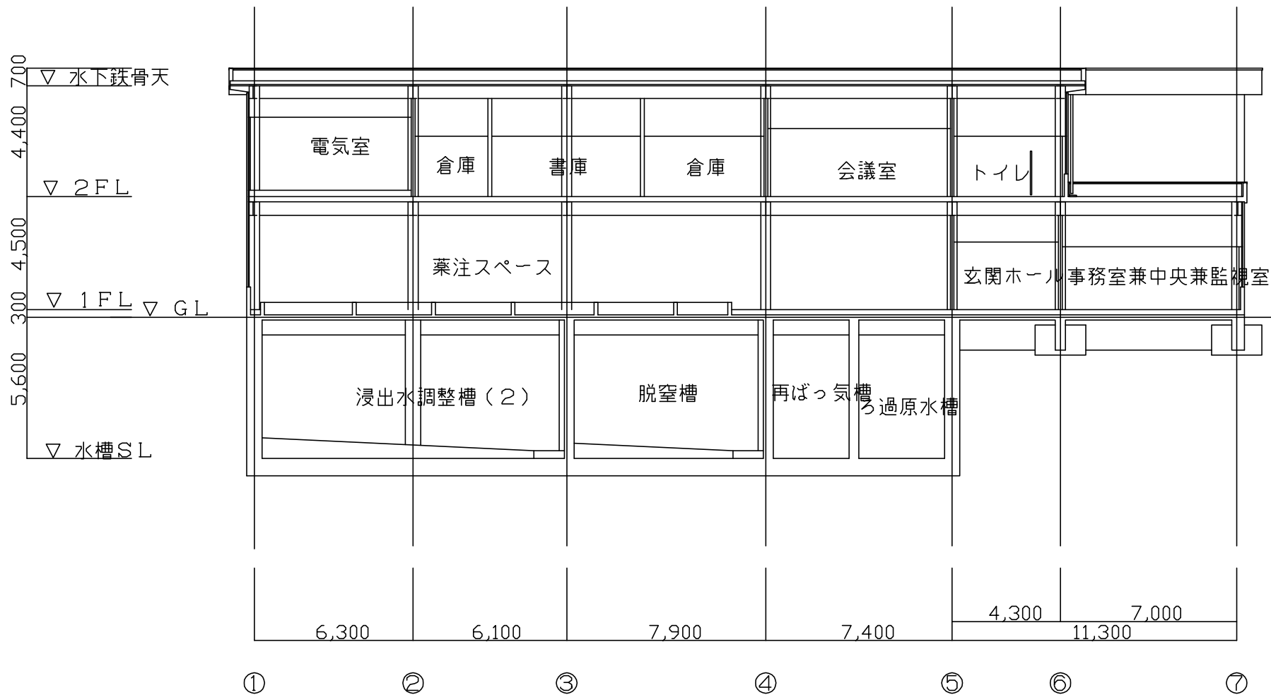
B-B断面図 S=1/150
