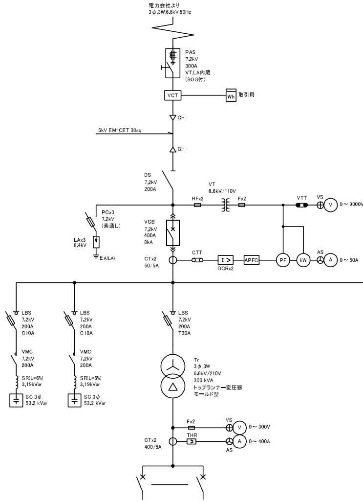
低圧動力盤 3φ,3W,200V
