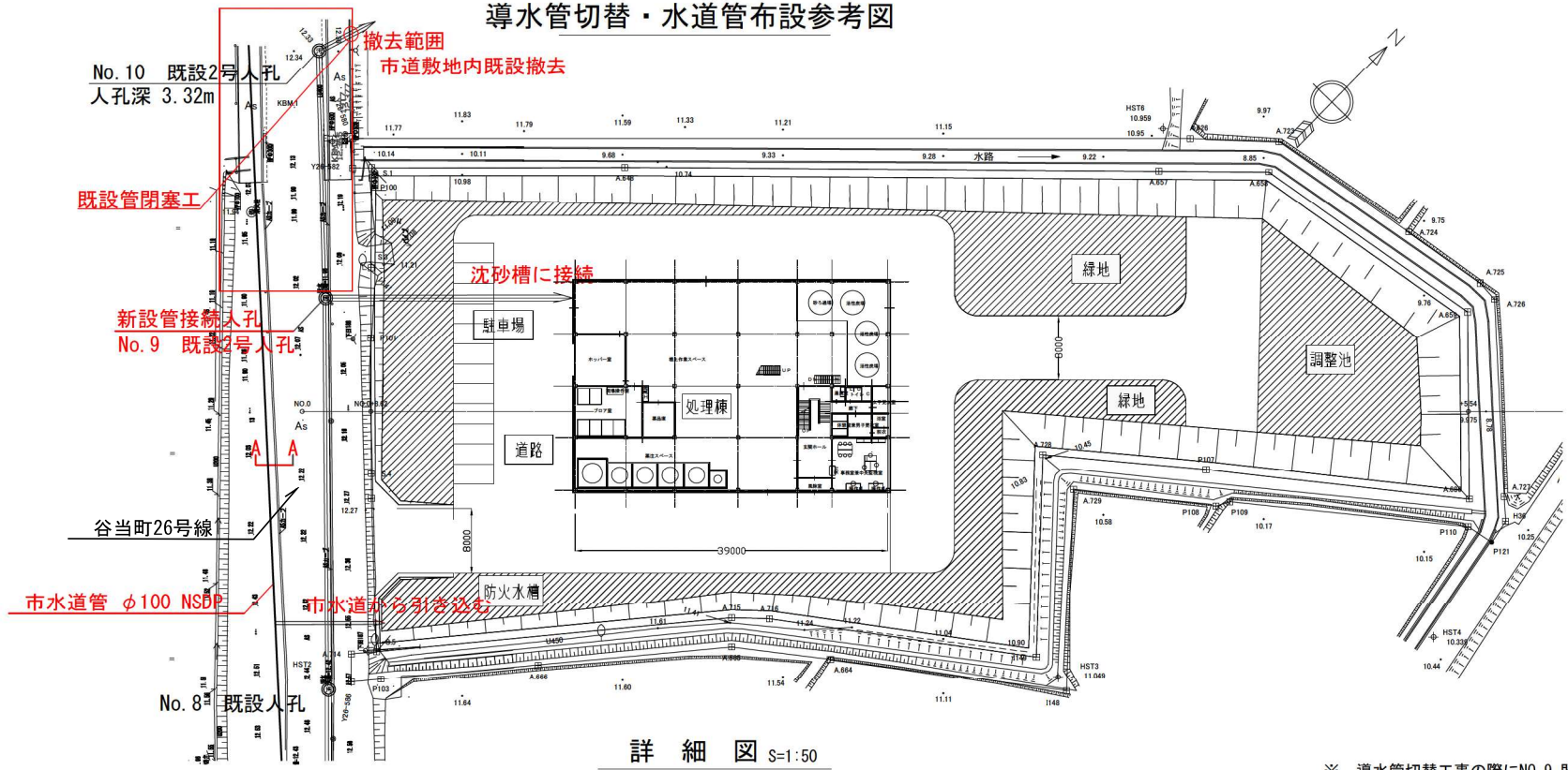
導水管切替詳細 平面図
