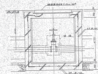
バルブポート詳細図 S=1/10
