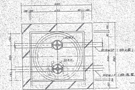
平面図 S=1/10
