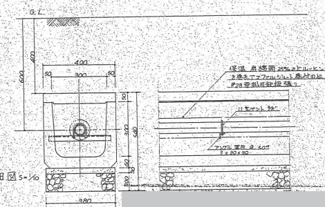
バルブポート詳細図 S=1/10
